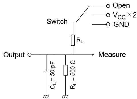
Fig. 11.7.1 AC Test Circuits
