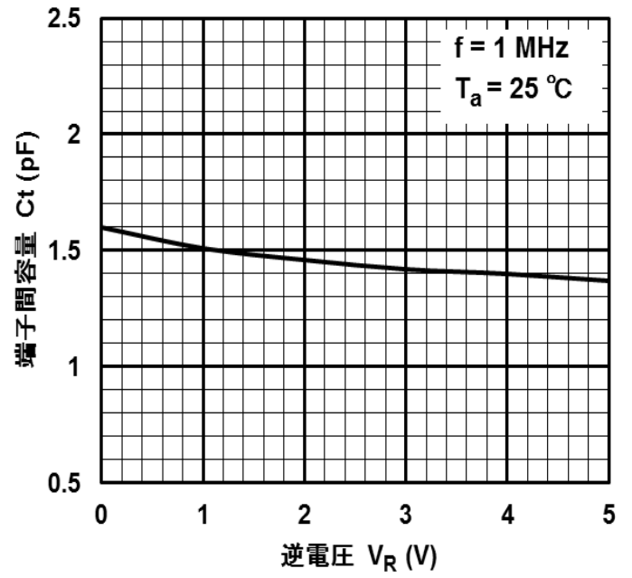
C_t - V_R
