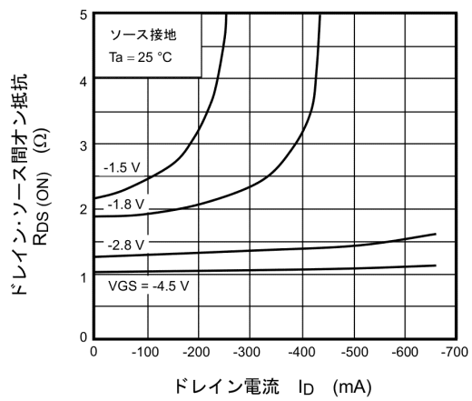
図 7.2.4 R_{DS(ON)} - I_D
