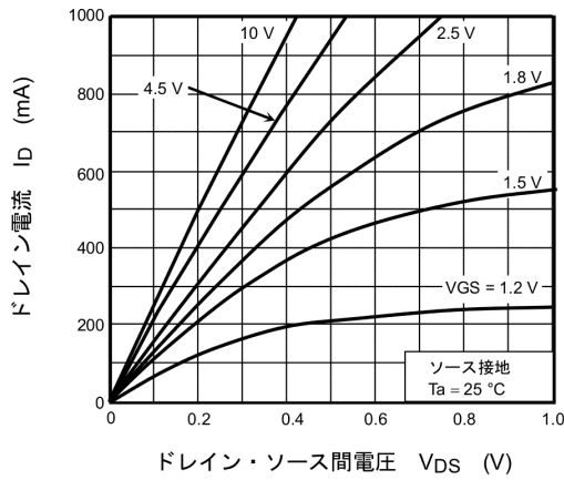
図 7.1.1 I_D - V_{DS}
