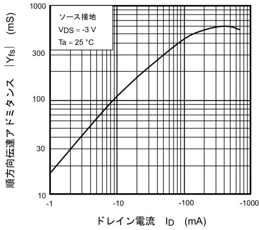
図 7.2.7 |Y_{fs}| - I_D
