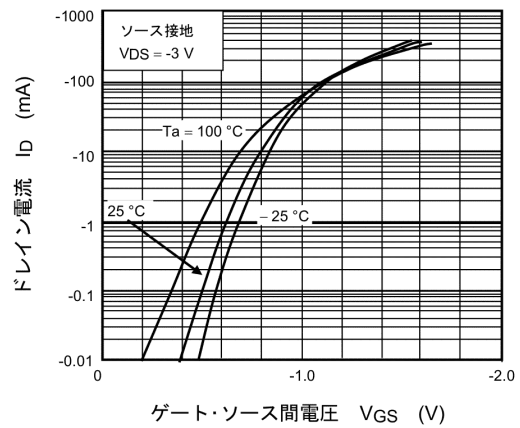
図 7.2.2 I_D - V_{GS}
