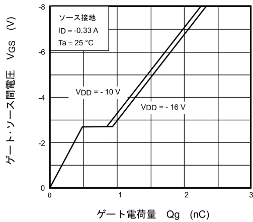
図 7.2.11 ダイナミック入力特性
