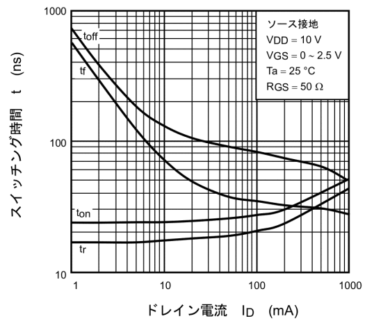
図 7.1.10 t - I_D
