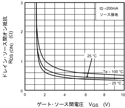
図 7.1.3 R_{DS(ON)} - V_{GS}
