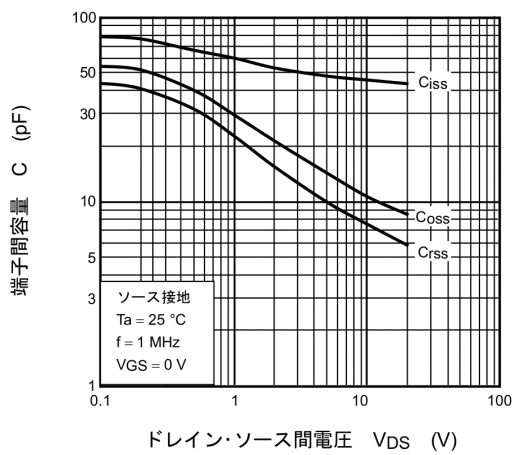
図 7.1.9 C - V_{DS}
