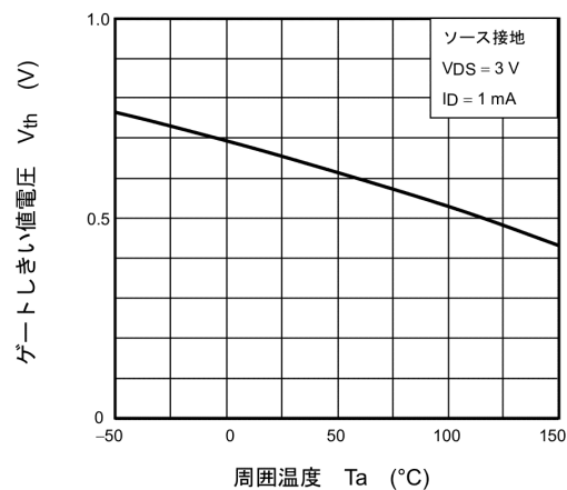
図 7.1.6 V_{th} - T_a
