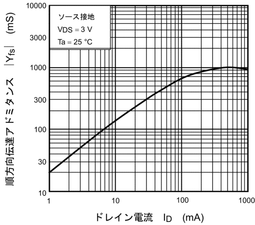
図 7.1.7 |Y_{fs}| - I_D
