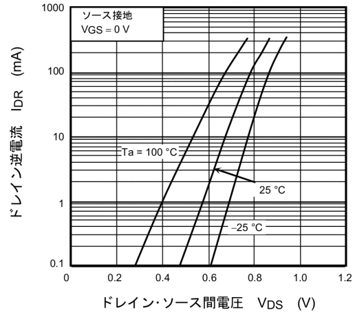
図 7.2.8 I_{DR} - V_{DS}
