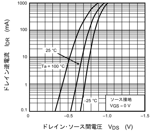
図 7.1.8 I_{DR} - V_{DS}
