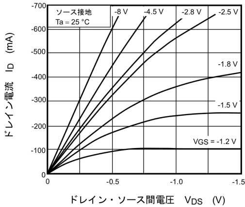
図 7.2.1 I_D - V_{DS}
