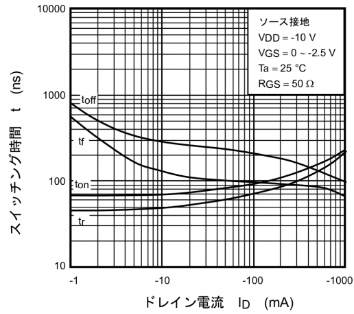
図 7.2.10 t - I_D
