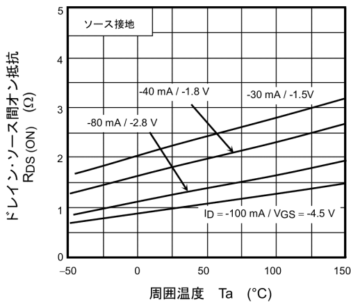
図 7.2.5 R_{DS(ON)} - T_a
