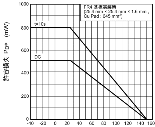
図 7.3.1 P_D - T_a
