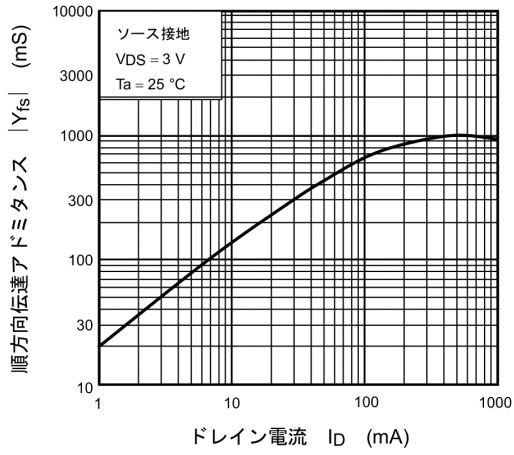
図 7.1.7 |Y_{fs}| - I_D
