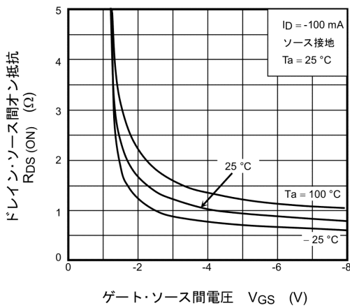
図 7.2.3 R_{DS(ON)} - V_{GS}
