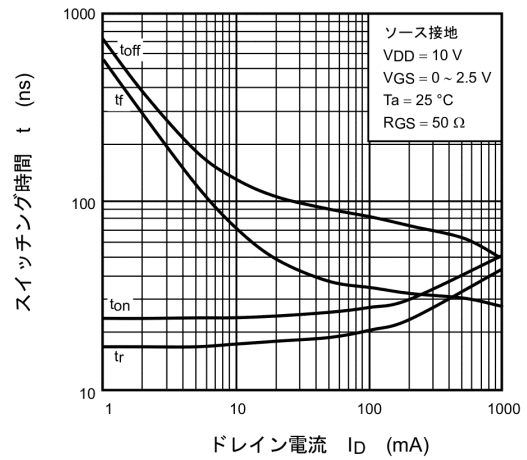
図 7.1.10 t - I_D
