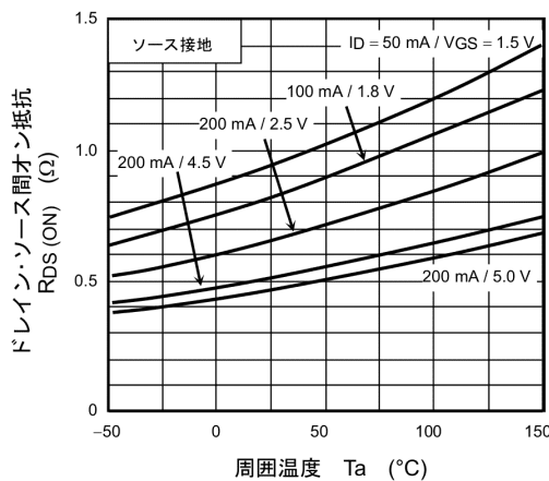
図 7.1.5 R_{DS(ON)} - T_a
