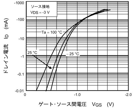
図 7.2.2 I_D - V_{GS}
