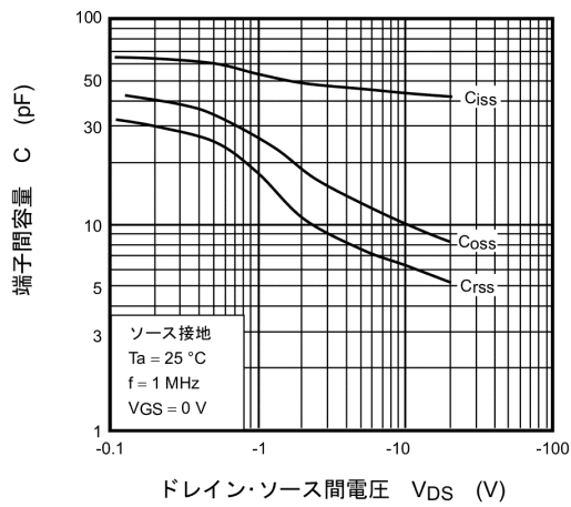
図 7.2.9 C - V_{DS}
