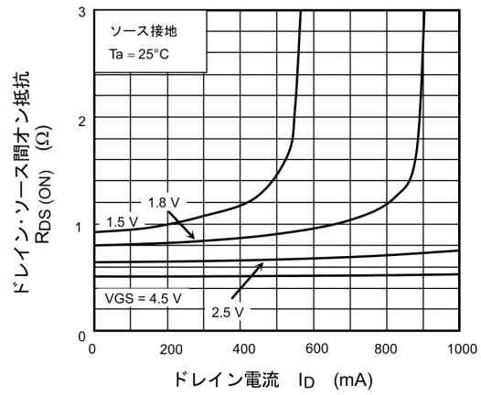
図 7.1.4 R_{DS(ON)} - I_D
