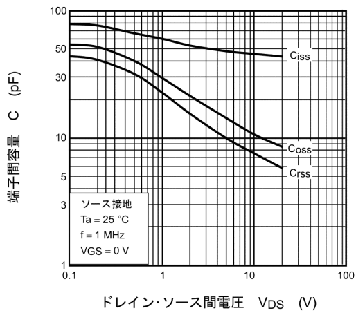
図 7.1.9 C - V_{DS}
