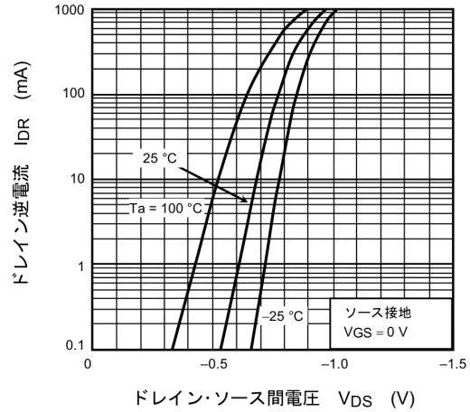
図 7.1.8 I_{DR} - V_{DS}
