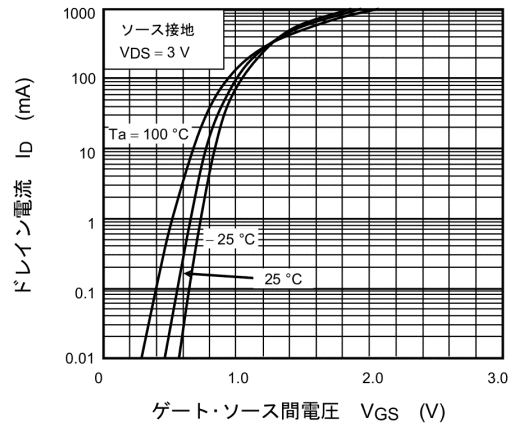
図 7.1.2 I_D - V_{GS}
