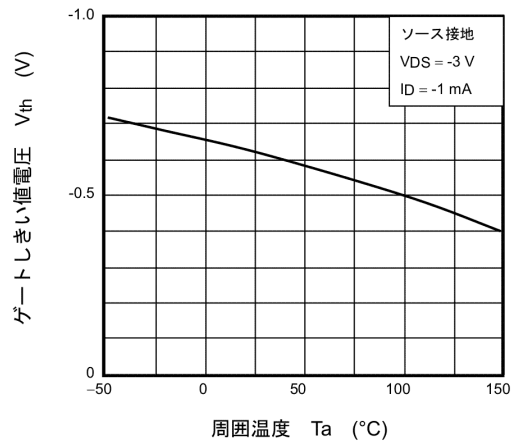
図 7.2.6 V_{th} - T_a
