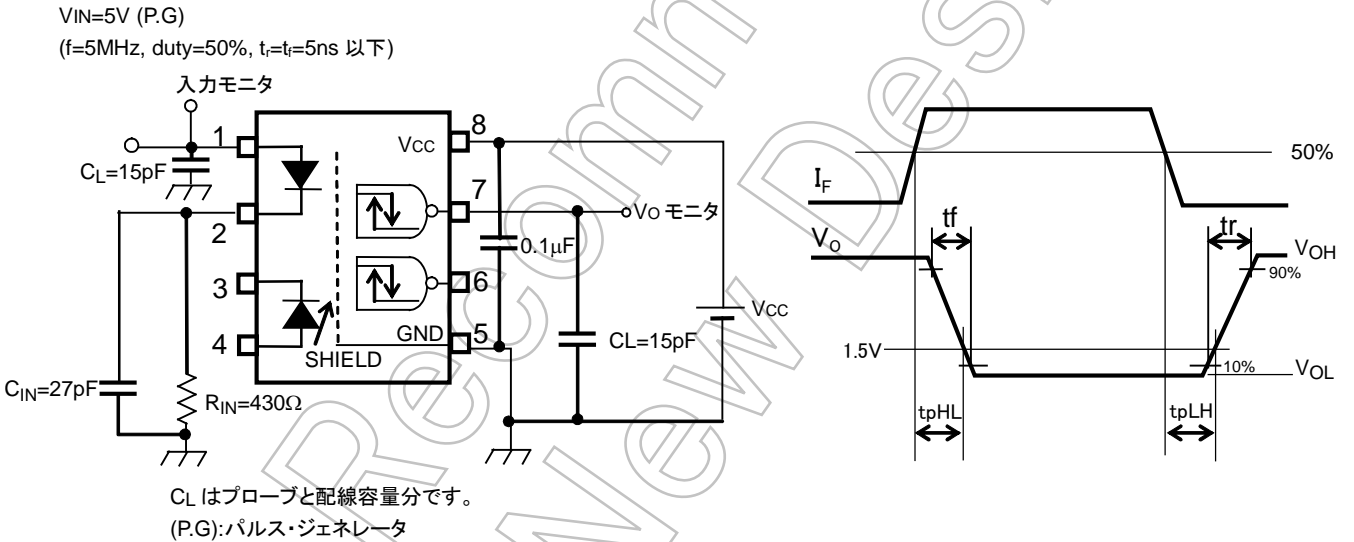
図 2 伝達遅延時間測定回路、波形
