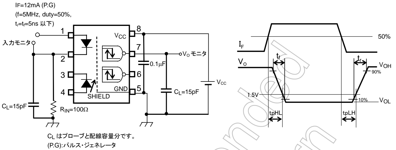
図 1 伝達遅延時間測定回路、波形
