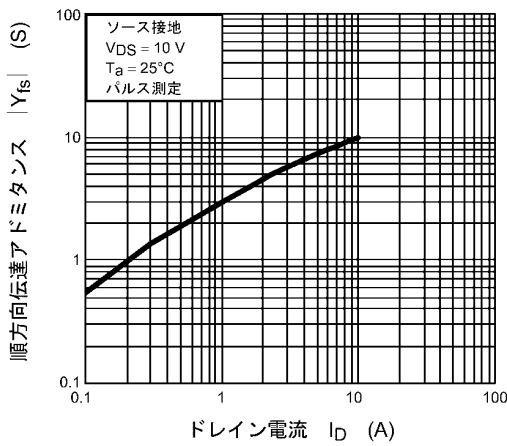
図 8.5 |Y_{fs}| - I_D
