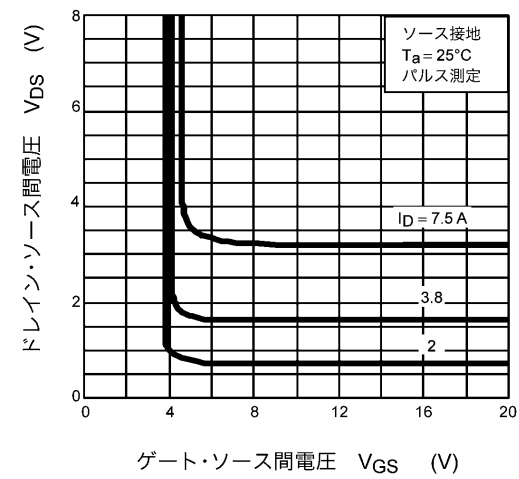
図 8.4 V_{DS} - V_{GS}
