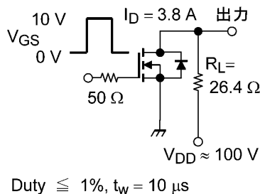
図 6.2.1 スイッチング時間の測定回路例
