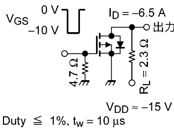
図 6.2.1 スwitching時間の測定回路例
