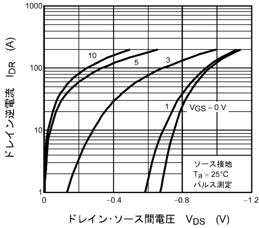
図 9.7 I_{DR} - V_{DS}
