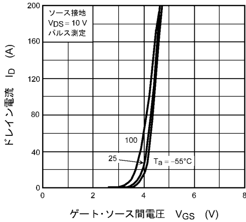
図 9.3 I_D - V_{GS}
