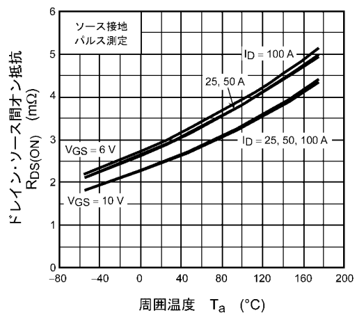
図 9.6 R_{DS(ON)} - T_a
