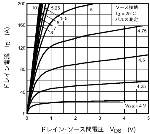
図 9.2 I_D - V_{DS}
