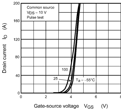
Fig. 9.3 I_D - V_{GS}
