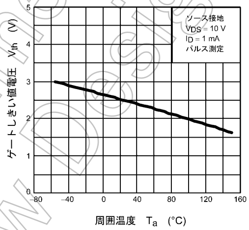
図 8.10 V_{th} - T_a
