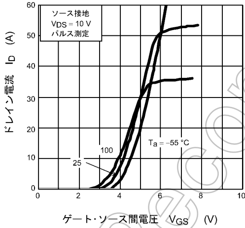
図 8.3 I_D - V_{GS}
