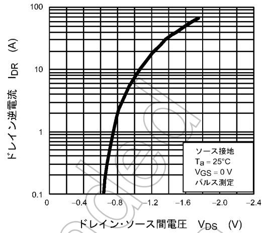
図 8.8 I_{DR} - V_{DS}
