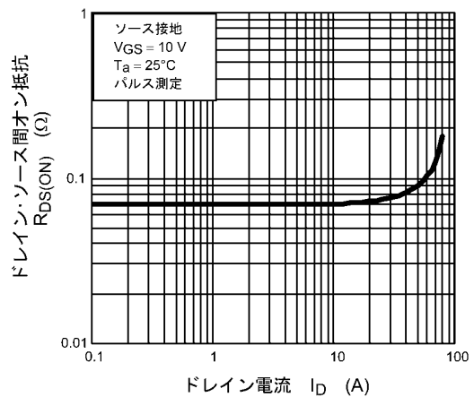
図 8.6 R_{DS(ON)} - I_D
