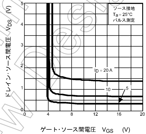
図 8.4 V_{DS} - V_{GS}
