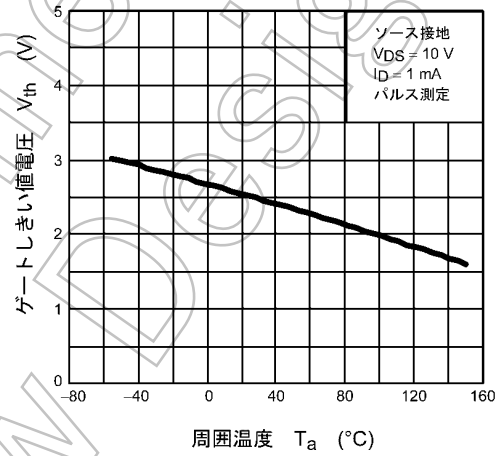
図 8.10 V_{th} - T_a
