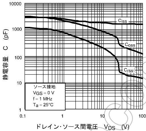
図 8.9 C - V_{DS}
