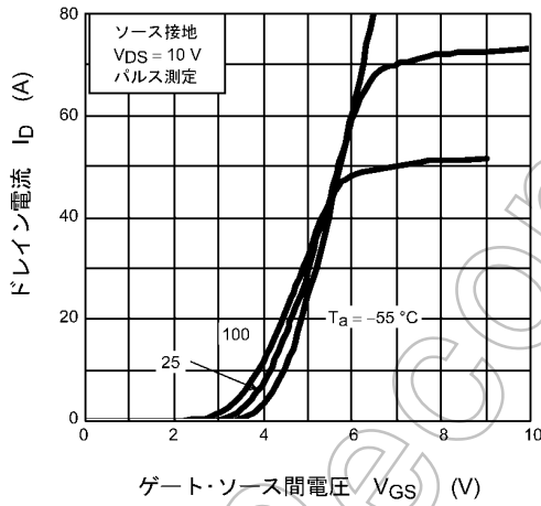
図 8.3 I_D - V_{GS}
