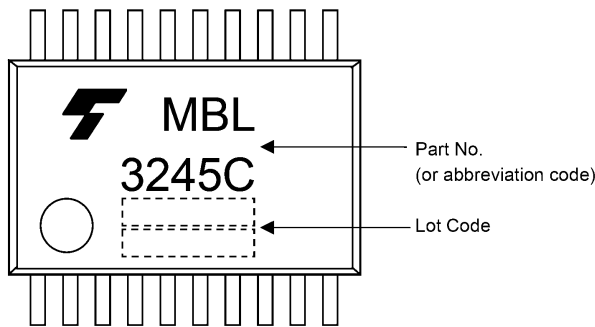
図 6.1 TSSOP20B
