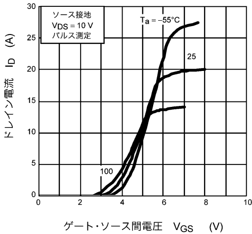
図 8.3 I_D - V_{GS}
