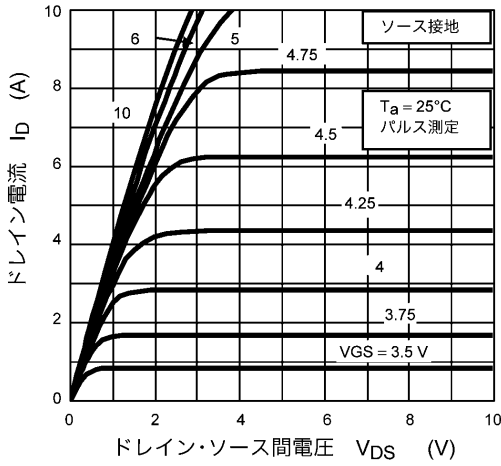
図 8.1 I_D - V_{DS}
