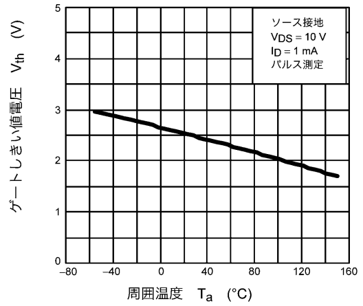
図 8.10 V_{th} - T_a
