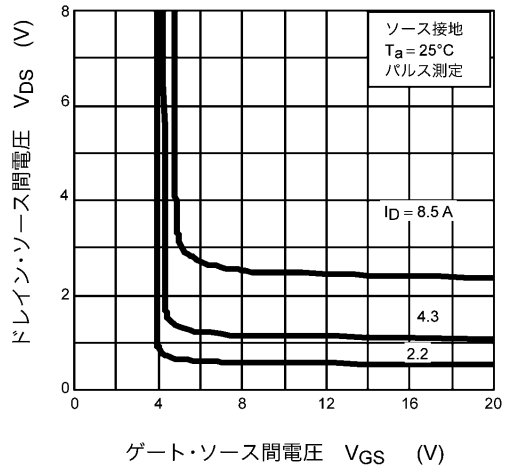
図 8.4 V_{DS} - V_{GS}
