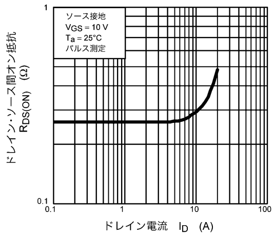
図 8.6 R_{DS(ON)} - I_D
