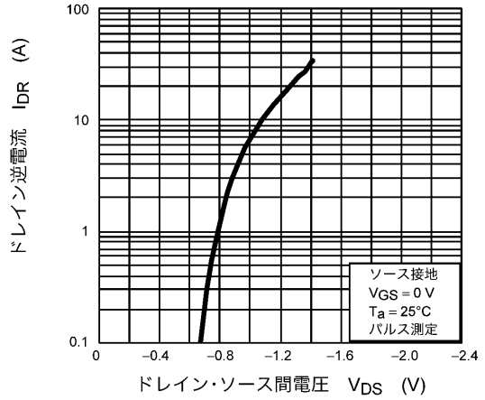
図 8.8 I_{DR} - V_{DS}
