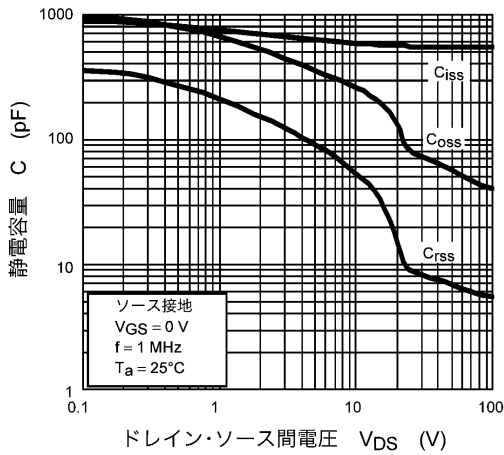
図 8.9 C - V_{DS}
