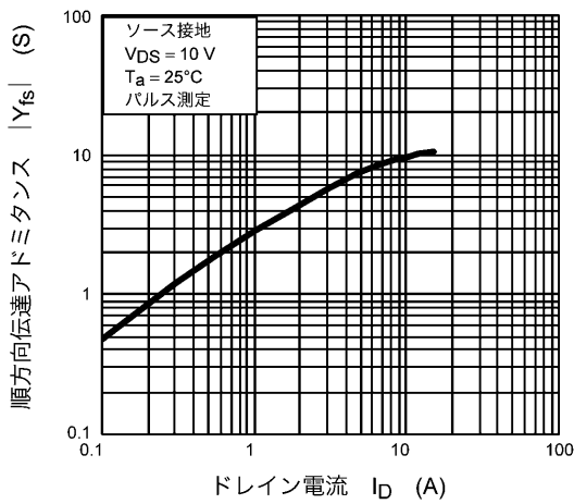
図 8.5 |Y_{fs}| - I_D
