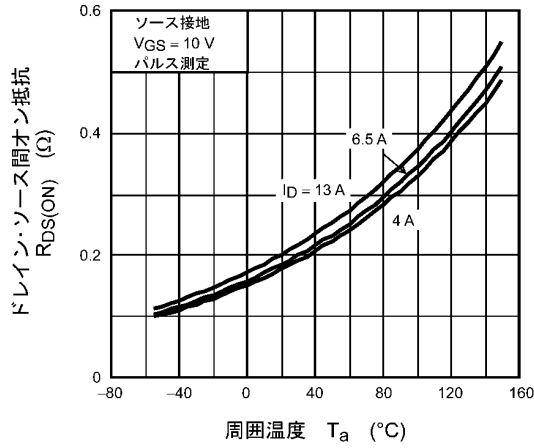
図 8.7 R_{DS(ON)} - T_a
