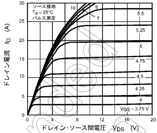
図 8.2 I_D - V_{DS}
