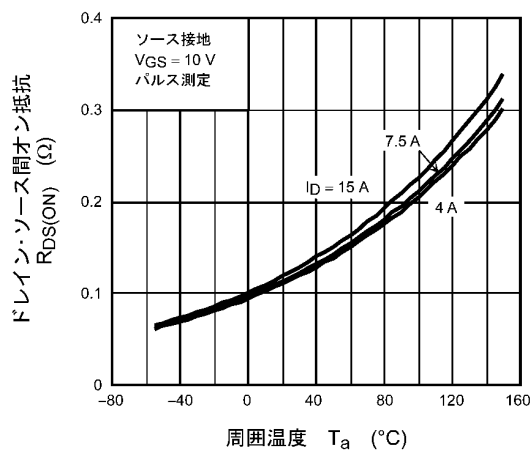
図 8.7 R_{DS(ON)} - T_a
