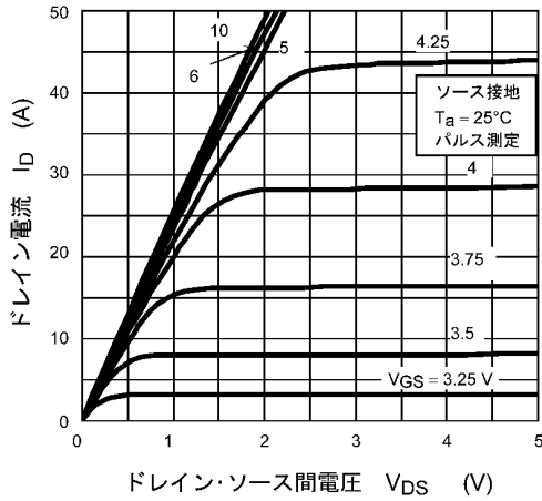
図 8.1 I_D - V_{DS}
