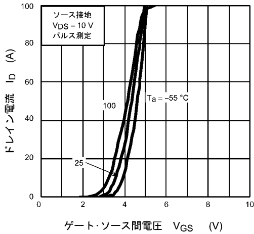
図 8.3 I_D - V_{GS}
