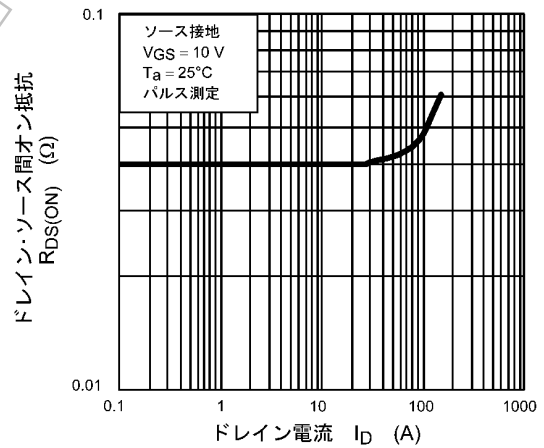
図 8.6 R_{DS(ON)} - I_D
