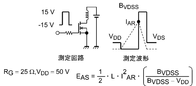
図 8.16 測定回路/測定波形
