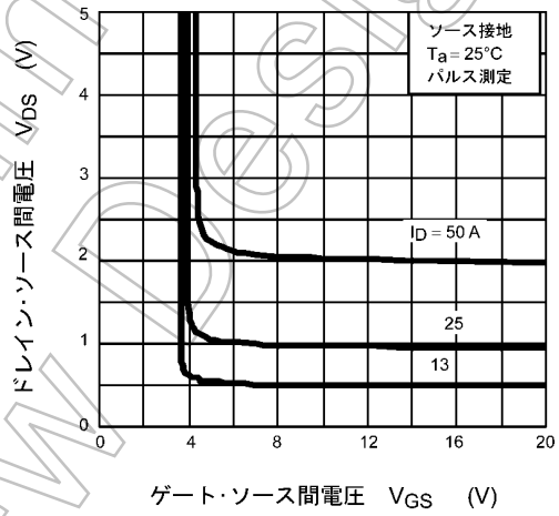
図 8.4 V_{DS} - V_{GS}
