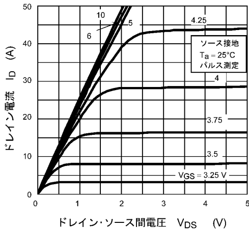
図 8.1 I_D - V_{DS}
