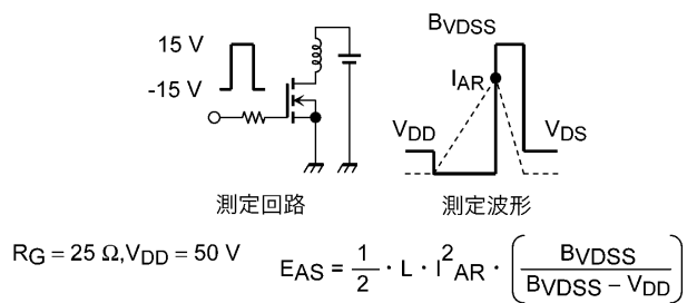
図 8.16 測定回路/測定波形
