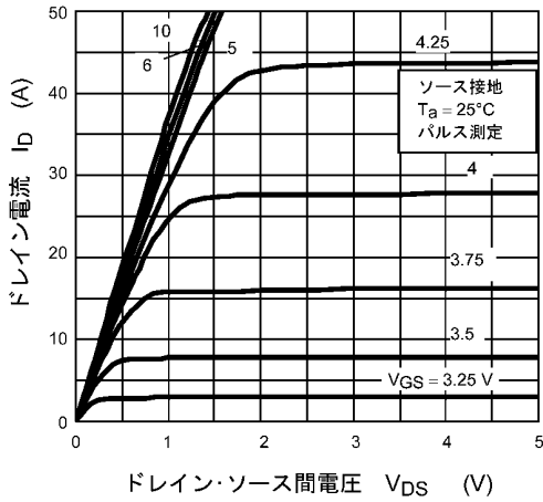
図 8.1 I_D - V_{DS}
