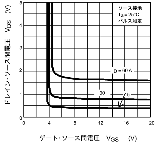
図 8.4 V_{DS} - V_{GS}
