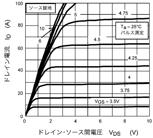
図 8.2 I_D - V_{DS}
