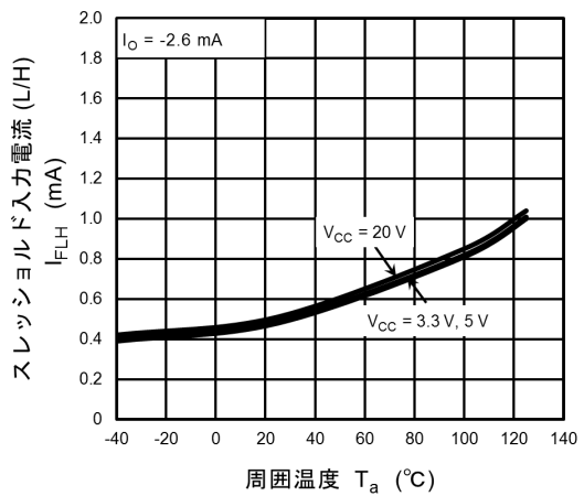
図 12.2.11 I_{FLH} - T_a
