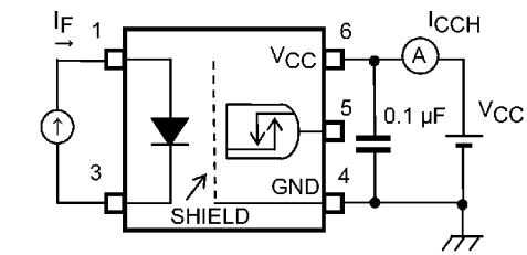
図 12.1.4 ICCH測定回路
