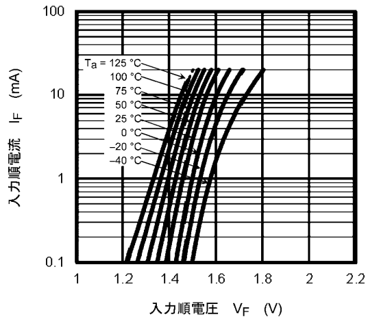
図 12.2.1 I_F - V_F
