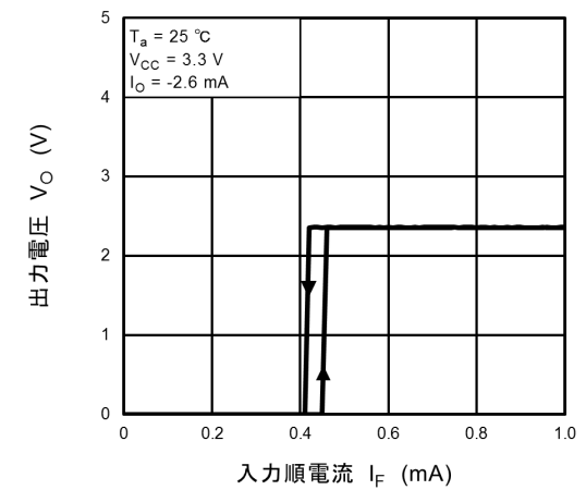
図 12.2.12 V_O - I_F
