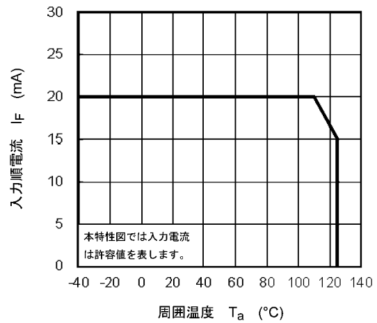
図 12.2.2 I_F - T_a
