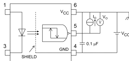
Fig. 12.1.2 VOH Test Circuit
