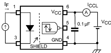
図 12.1.3 ICCL測定回路
