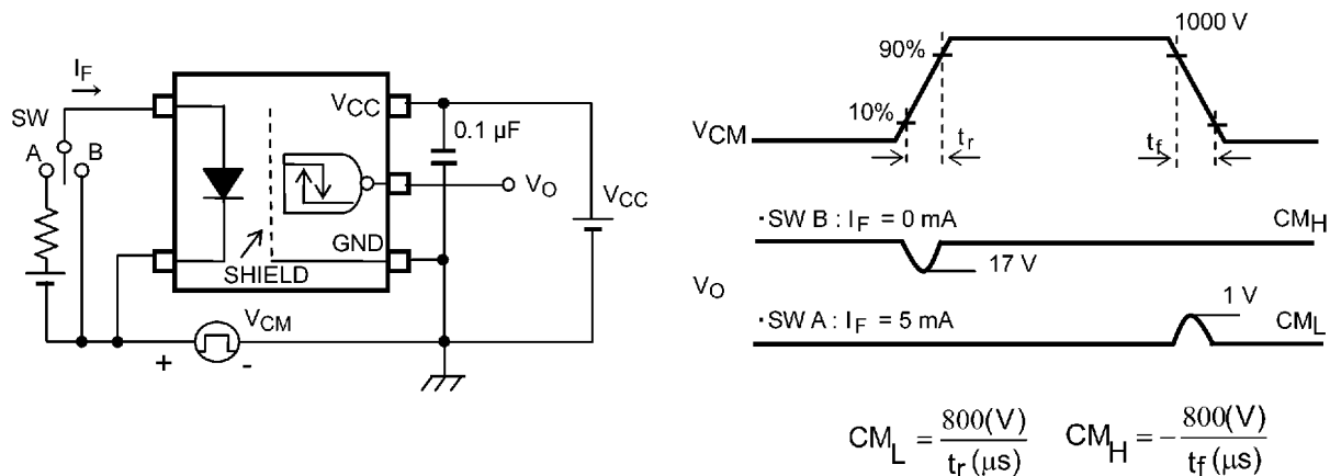
図 12.1.8 コモンモード過渡耐性測定回路, 波形
