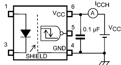
図 12.1.4 ICCH測定回路
