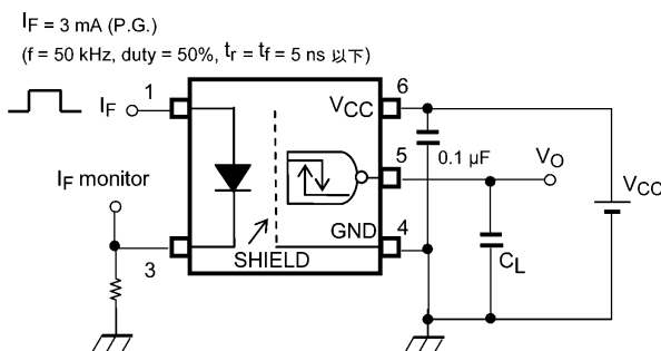
図 12.1.5 IOSL測定回路
