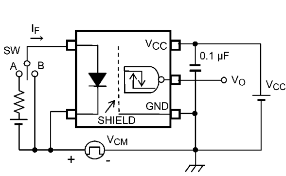
図 12.1.8 コモンモード過渡耐性測定回路, 波形
