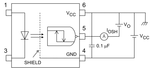
図 12.1.6 I OSH 測定回路
