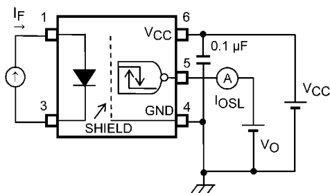
図 12.1.5 IOSL測定回路
