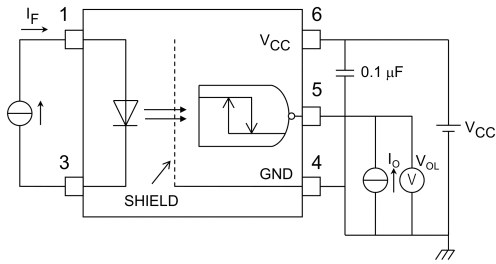
図 12.1.1 V OL 測定回路
