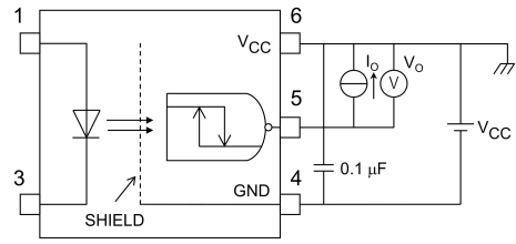
図 12.1.2 V OH 測定回路
