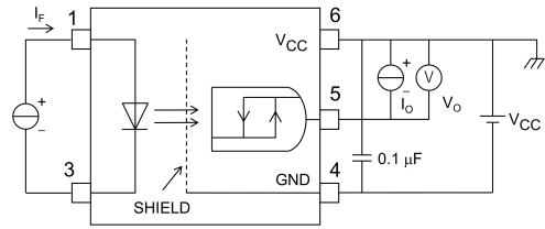
Fig. 12.1.2 V_{OH} Test Circuit
