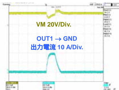
OUT1 地絡波形 OUT1-GND
