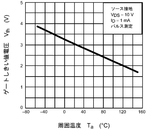
図 8.10 V_{th} - T_a
