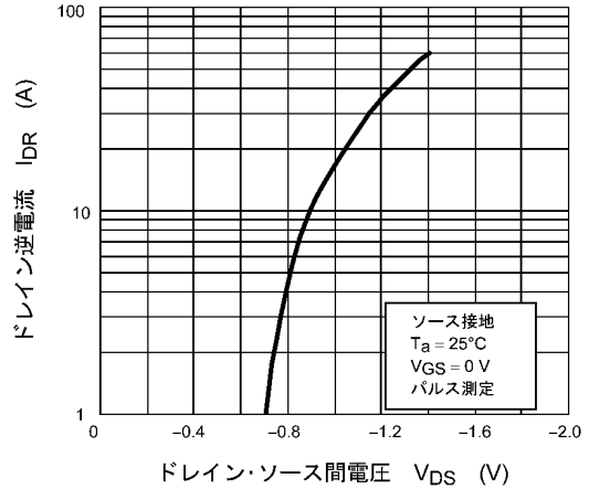
図 8.8 I_{DR} - V_{DS}
