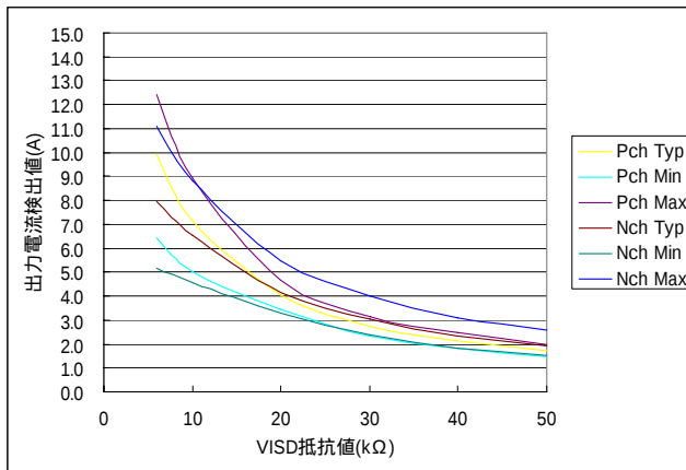
VISD 端子の外付け抵抗値 – ISD 検出電流値の関係 (参考値)
