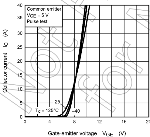
Fig. 8.5 I_C - V_{GE}
