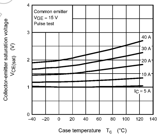
Fig. 8.6 V_{CE(\text{sat})} - T_c
