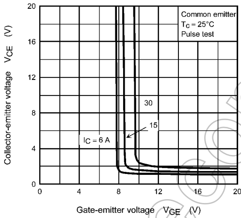
Fig. 8.3 V_{CE} - V_{GE}
