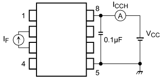
図 13.1.5 ICCH測定回路
