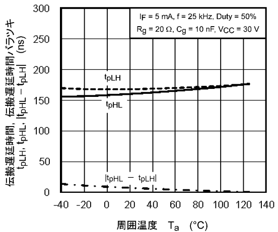
図 13.2.12 t_{pLH}, t_{pHL}, |t_{pHL} - t_{pLH}| - T_a
