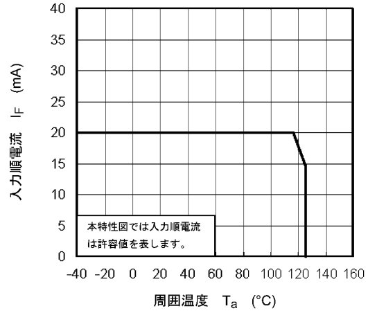
図 13.2.2 I_F - T_a
