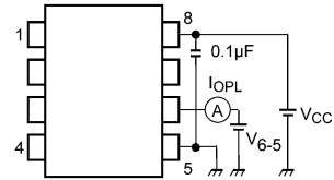
図 13.1.2 I OLP 測定回路
