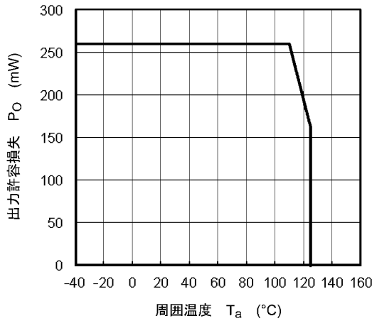
図 13.2.3 P_O - T_a
