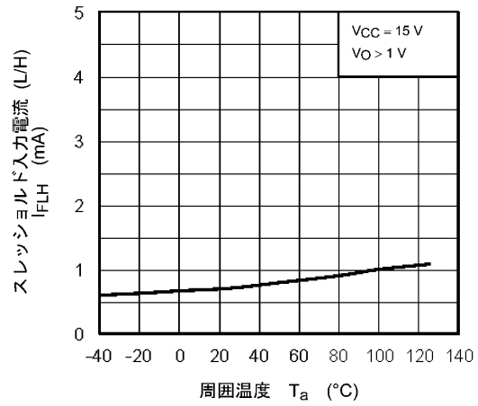
図 13.2.4 I_{FLH} - T_a
