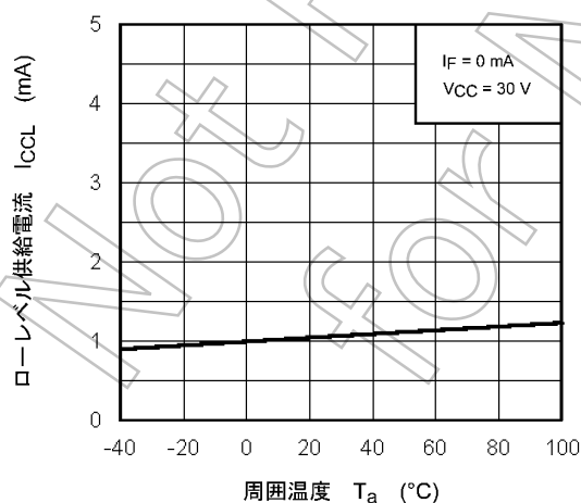
図 12.2.5 I_{cCL} - T_a
