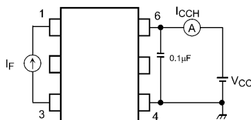
図 12.1.5 I CCH 測定回路
