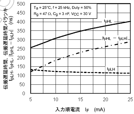
図 12.2.12 t_{pLH}, t_{pHL}, |t_{pHL} - t_{pLH}| - I_F
