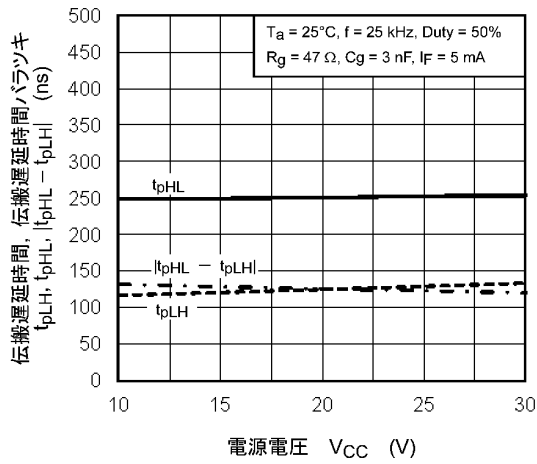
図 12.2.13 t_{pLH}, t_{pHL}, |t_{pHL} - t_{pLH}| - V_{CC}
