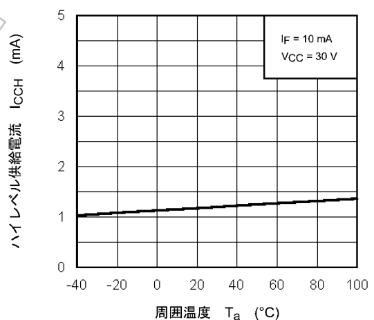
図 12.2.6 I_{cCH} - T_a
