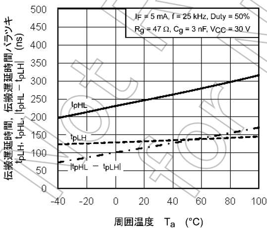
図 12.2.11 t_{pLH}, t_{pHL}, |t_{pHL} - t_{pLH}| - T_a
