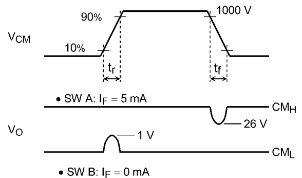
図 12.1.8 コモンモード過渡耐性測定回路, 波形
