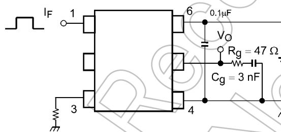
図 12.1.7 伝搬遅延時間測定回路, 波形
