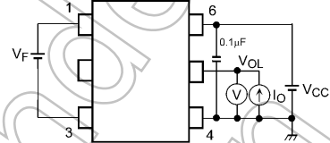
図 12.1.2 I OPL 測定回路
