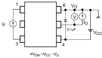
図 12.1.3 V OH 測定回路
