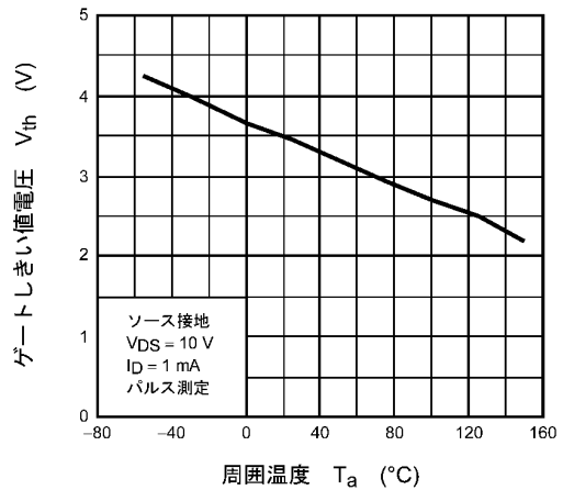
図 8.10 V_{th} - T_a
