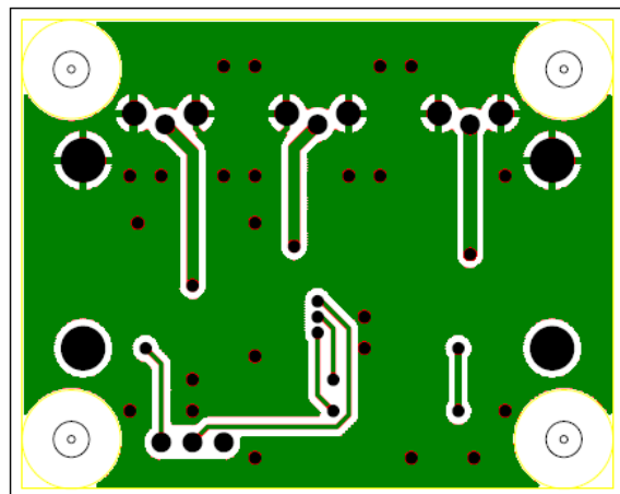
半田面パターン
