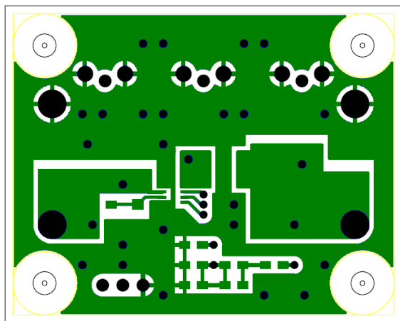
部品面パターン
