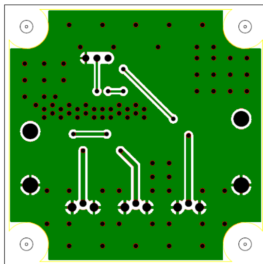
半田面パターン
