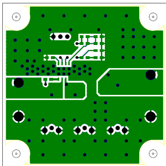
部品面パターン
