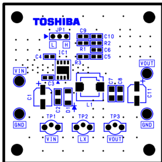
部品面シルク
