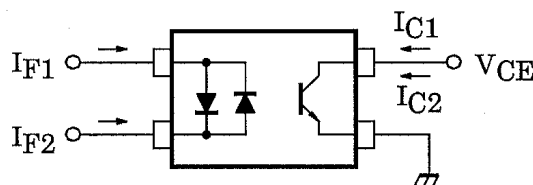
図 8.1 コレクタ電流比測定回路
