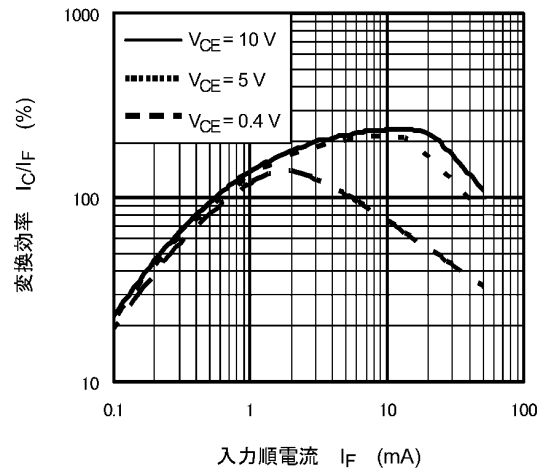
図 11.11 I_C/I_F - I_F
