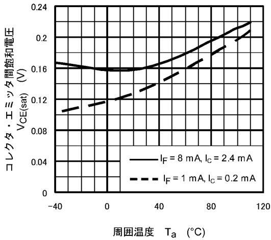
図 11.12 V_{CE(sat)} - T_a
