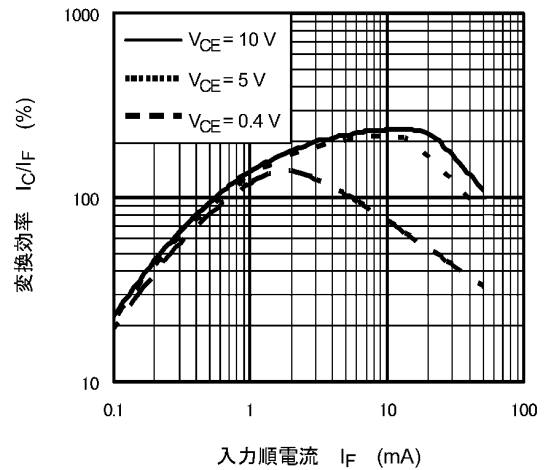
図 11.11 I_C/I_F - I_F
