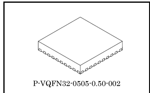
TB6569FTG:質量: 0.07 g (標準)
