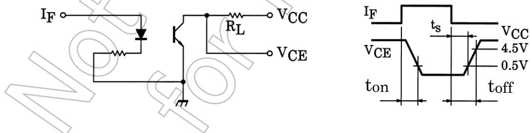
図 1: スwitchング時間測定回路
