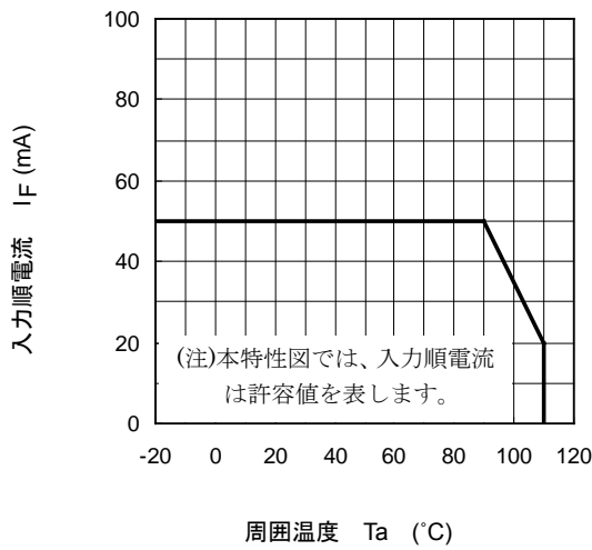
I_F - T_a
