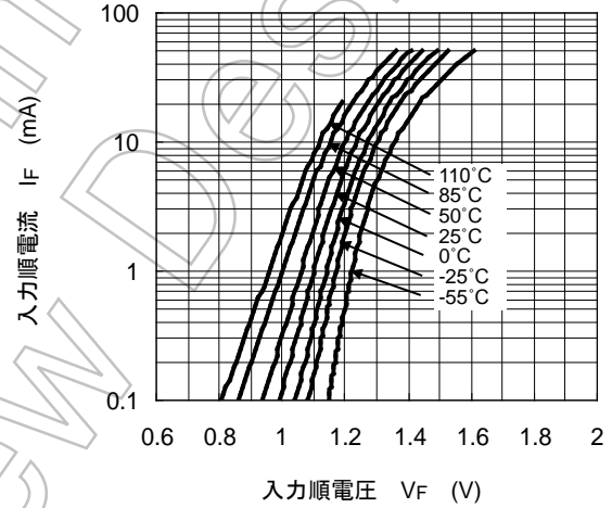
I_{FP} - V_{FP}
