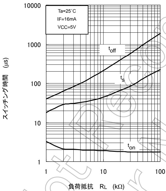
スイッチング時間 - R_L
