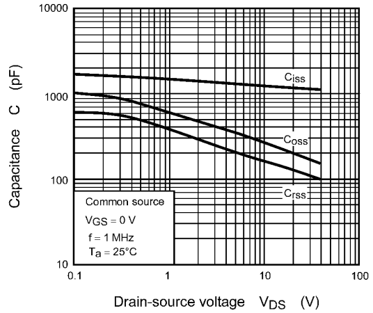
Fig. 8.8 Capacitance - V_{DS}
