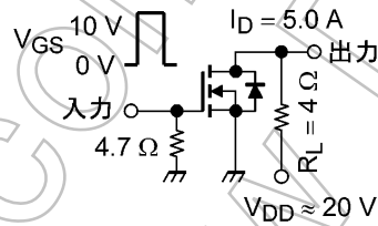
図 6.2.1 スwitching時間の測定回路例
