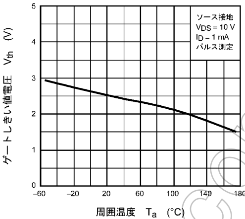
図 8.9 V_{th} - T_a (注7)
