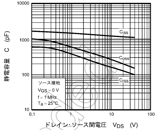
図 8.8 静電容量 - V_{DS}
