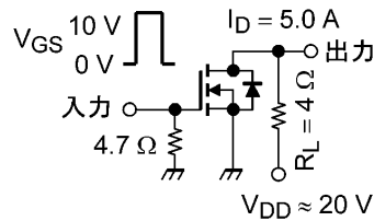
図 6.2.1 スwitchング時間の測定回路例
