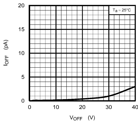
Fig. 12.1.10 I_{OFF} - V_{OFF}
