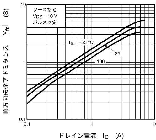
図 8.5 |Y_{fs}| - I_D
