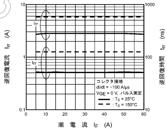
図 8.18 I_{rr} , t_{rr} - I_F
