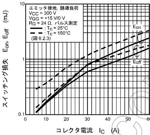
図 8.15 E_{on} , E_{off} - I_C
