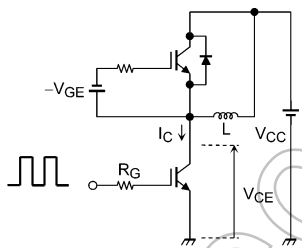
図 6.2.1 スwitchング時間の測定回路
