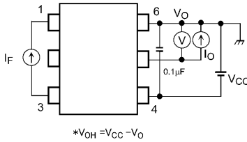
図 12.1.3 V OH 測定回路
