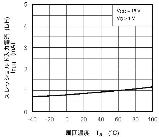
図 12.2.4 I_{FLH} - T_a
