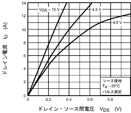
図 9.1 I_D - V_{DS}
