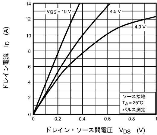
図 8.1 I_D - V_{DS}
