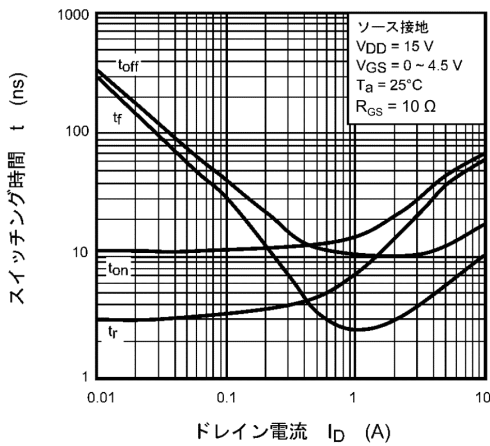
図 9.11 t - I_D
