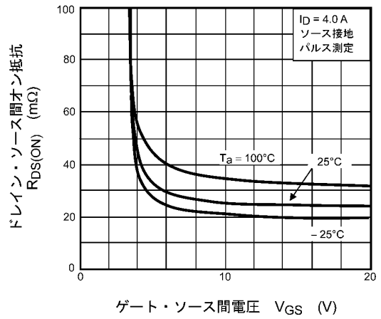
図 9.4 R_{DS(ON)} - V_{GS}
