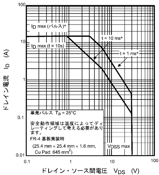
図 8.15 安全動作領域
