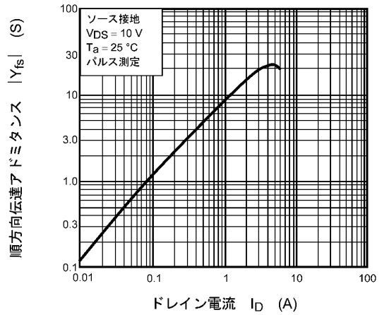
図 8.8 |Y_{fs}| - I_D
