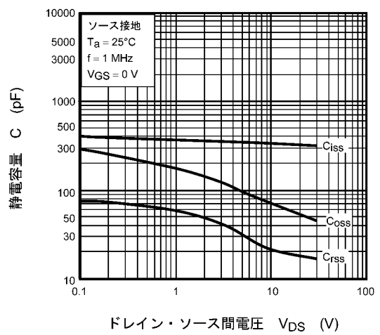
図 8.10 C - V_{DS}
