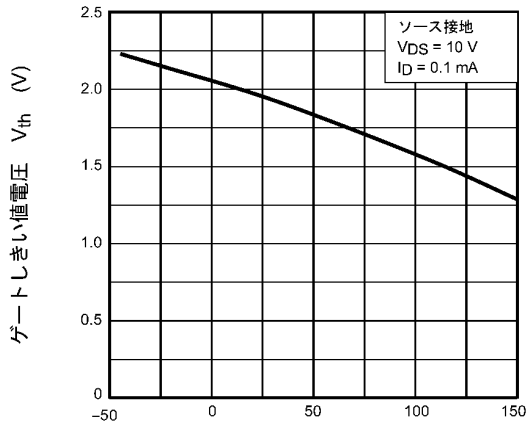
図 9.7 V_{th} - T_a
