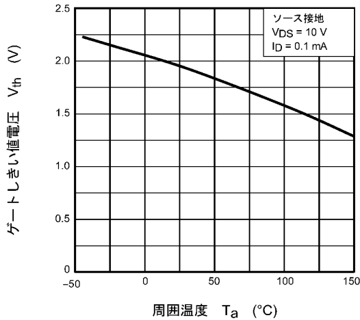
図 8.7 V_{th} - T_a
