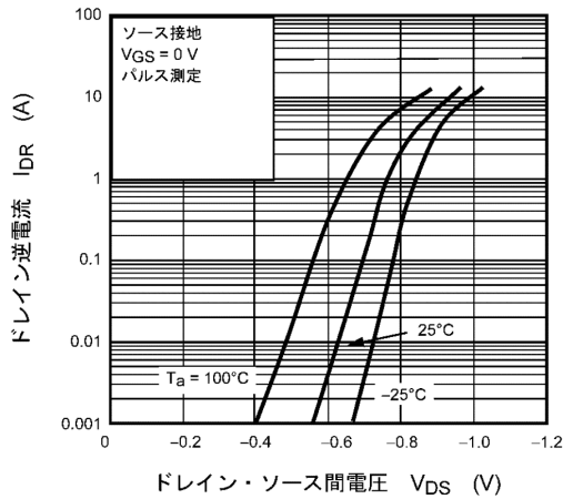
図 9.9 I_{DR} - V_{DS}
