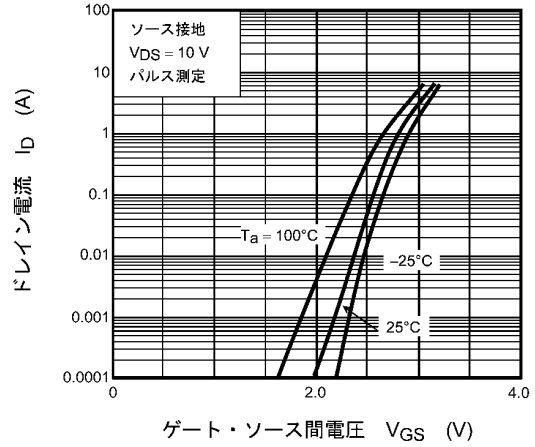
図 8.2 I_D - V_{GS}
