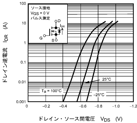
図 8.9 I_{DR} - V_{DS}
