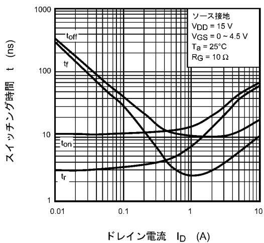
図 8.11 t - I_D
