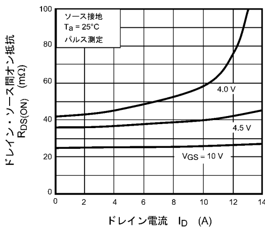
図 9.5 R_{DS(ON)} - I_D
