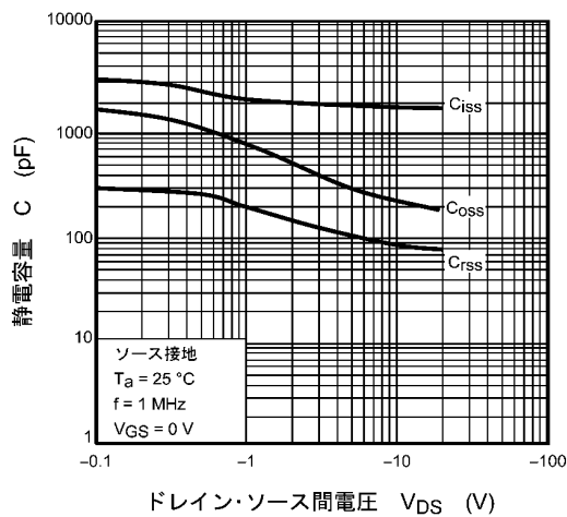
図 7.9 C - V_{DS}
