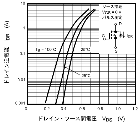
図 7.8 I_{DR} - V_{DS}
