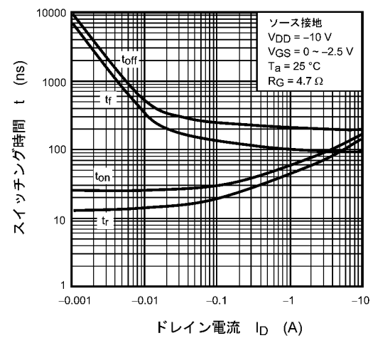
図 7.10 t - I_D
