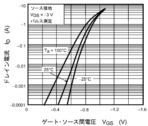
図 7.2 I_D - V_{GS}
