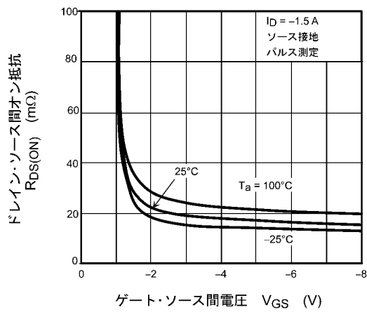
図 7.3 R_{DS(ON)} - V_{GS}
