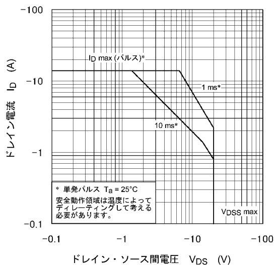
図 7.14 安全動作領域
