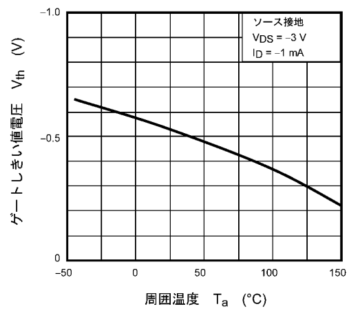
図 7.6 V_{th} - T_a
