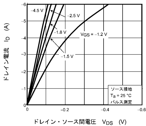
図 7.1 I_D - V_{DS}
