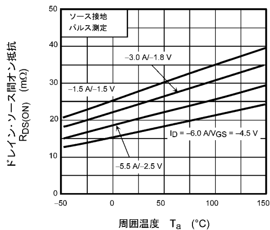
図 7.5 R_{DS(ON)} - T_a
