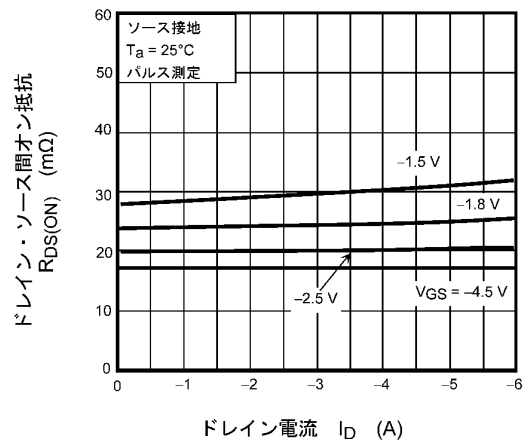
図 7.4 R_{DS(ON)} - I_D
