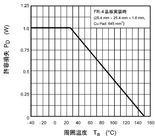
図 7.13 P_D - T_a
