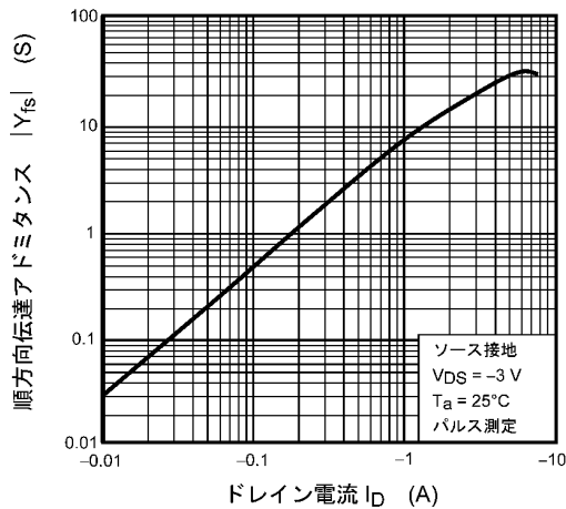
図 7.7 |Y_{fs}| - I_D
