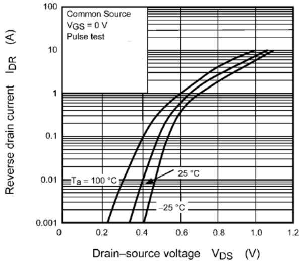
Fig. 7.9 I_{DR} - V_{DS}
