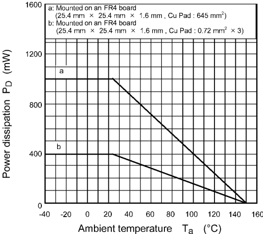
Fig. 7.13 P_D - T_a
