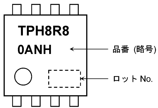
図 7.1 現品表示
