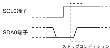
図 20-10 ストップコンディションの発生
