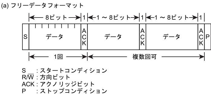
図 20-3 フリーデータフォーマット
