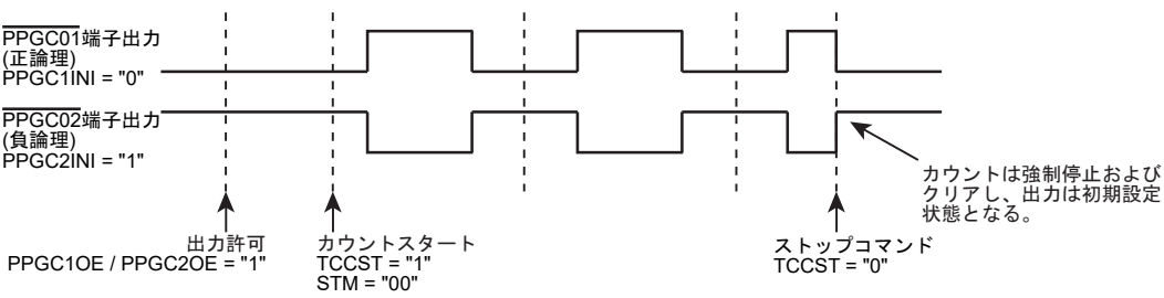
図 15-14 出力初期状態でカウント即時停止クリア (TC0CR3<STM> = “00”)
