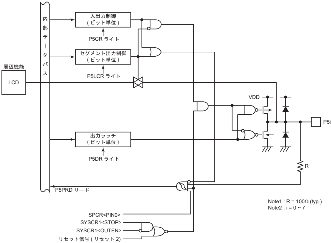
図 8-8 P5 ポート
