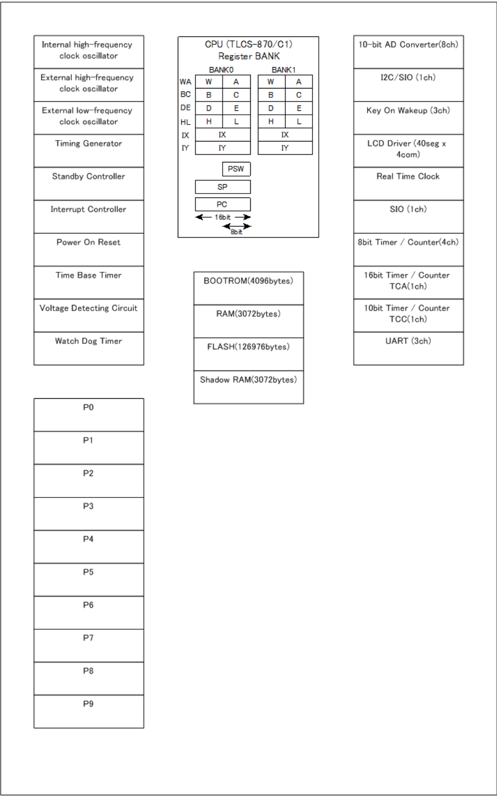
図 1-2 ブロック図
