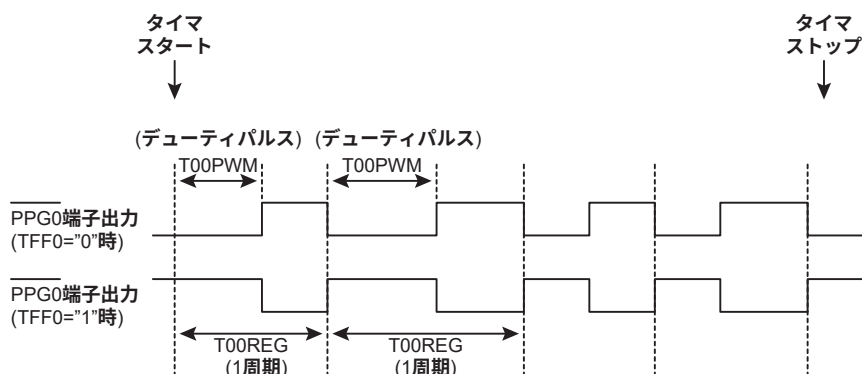
図 16-8 PPG0 パルス出力
