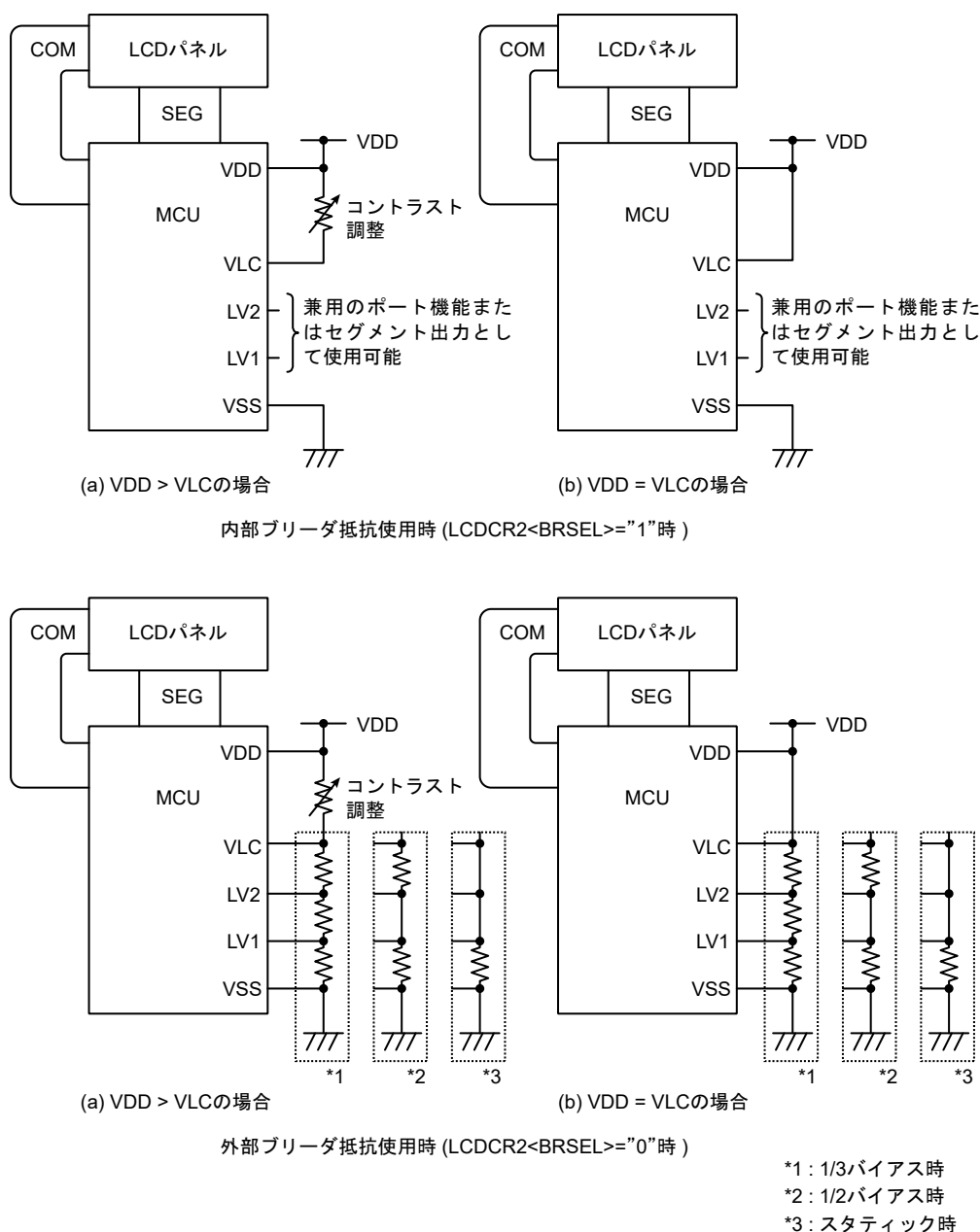
図 23-4 接続例
