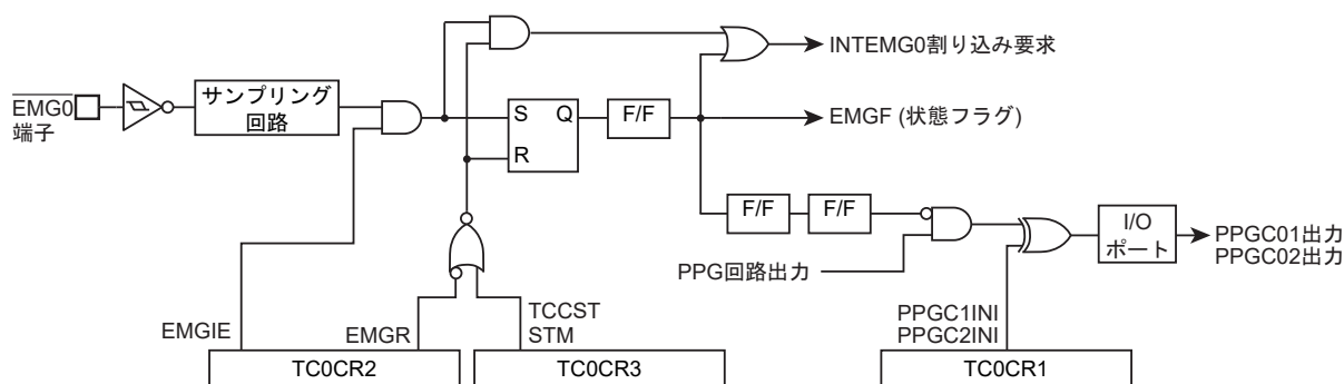
图 15-22 EMG0 端子
