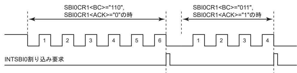
図 20-5 データ転送クロック数と SBI0CR1<BC>, SBI0CR1<ACK>
