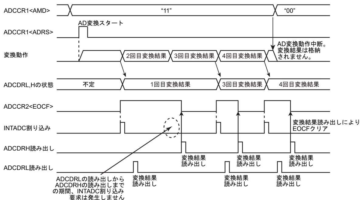
図 22-3 リピートモード
