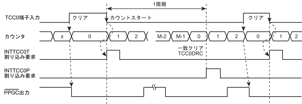
図 15-20 トリガスタート割り込み
