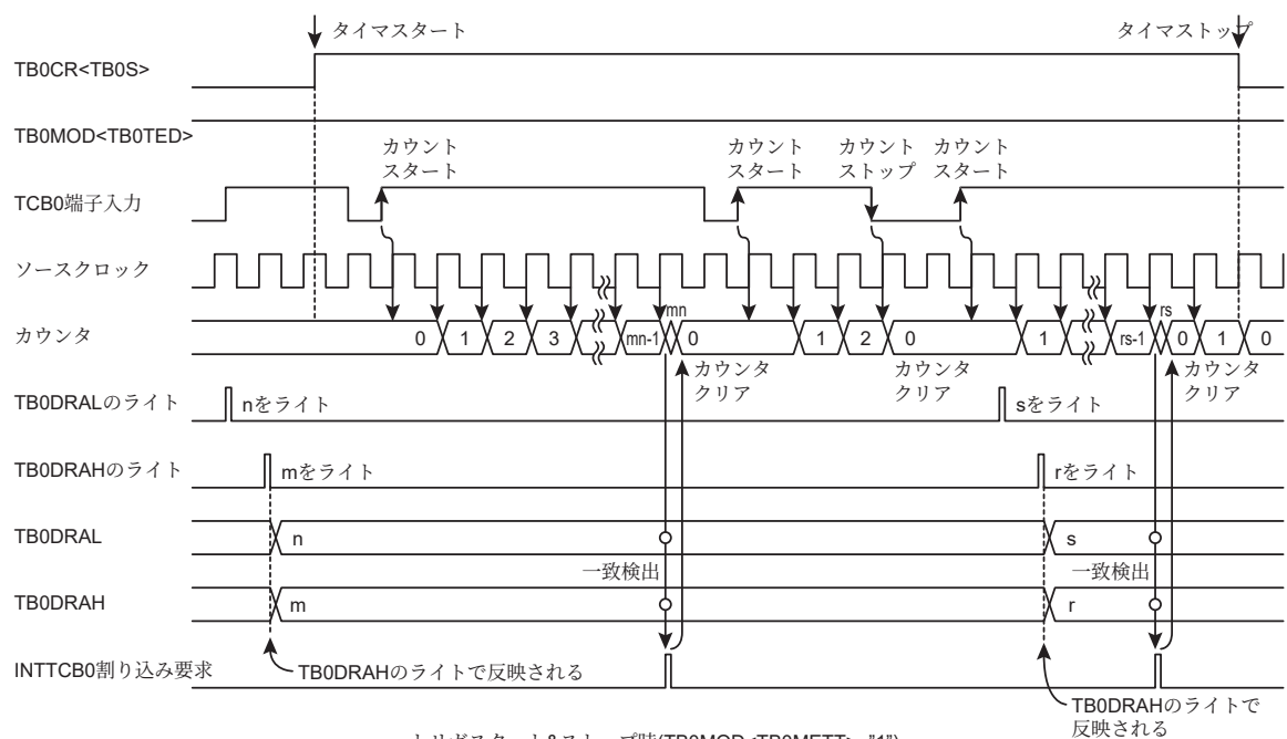
図 14-4 外部トリガタイミングチャート
