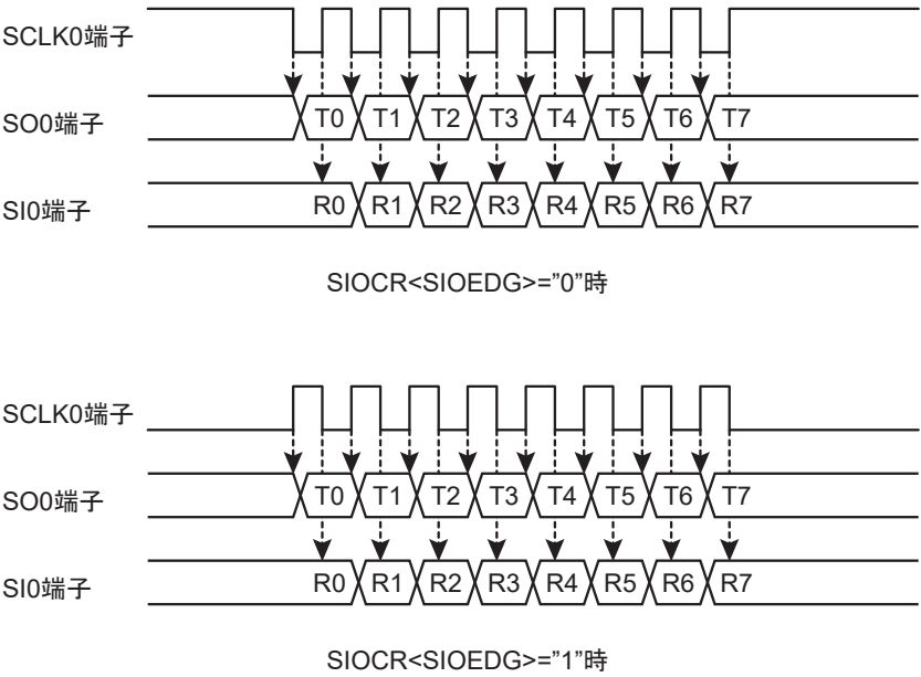
図 19-2 転送エッジ
