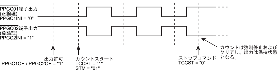
図 15-15 出力保持状態でカウント即時停止クリア (TC0CR3<STM> = “01”)
