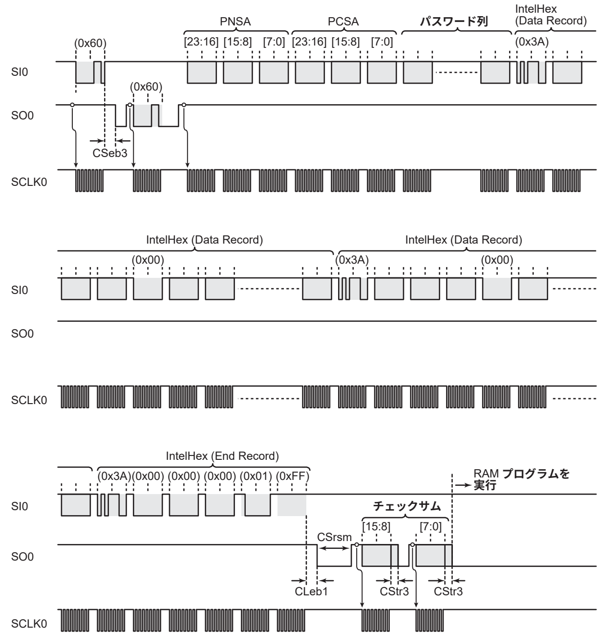
図 26-21 RAM ロードコマンド
