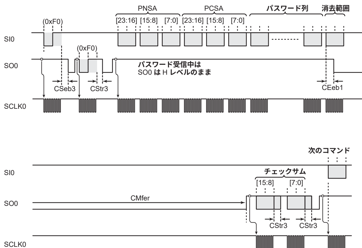
図 26-18 フラッシュメモリ消去コマンド
