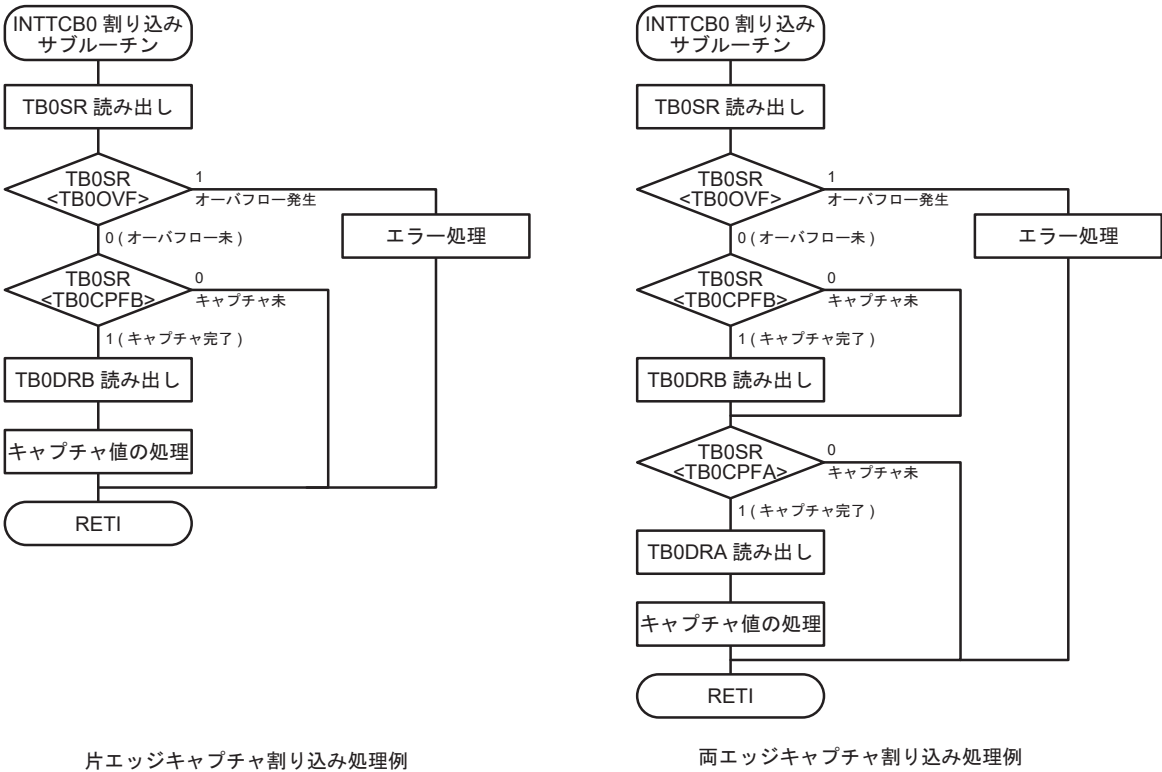
図 14-8 キャプチャ処理例
