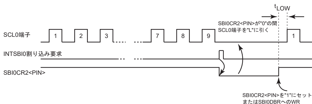
図 20-11 SBI0CR2<PIN>と SCL0 端子
