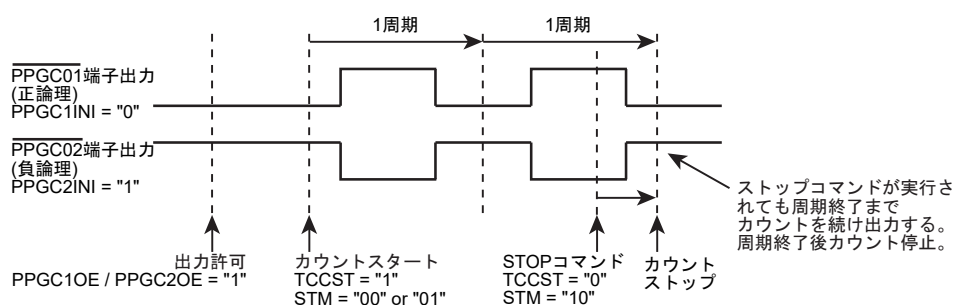
図 15-16 周期出力後カウント停止 (TC0CR3<STM> = “10”)
