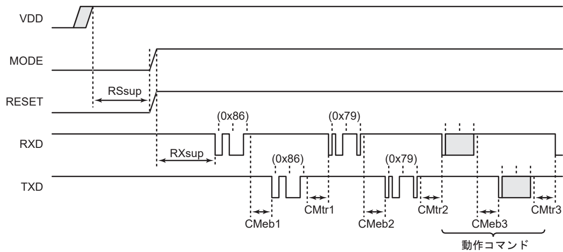
図 26-6 リセットタイミグ
