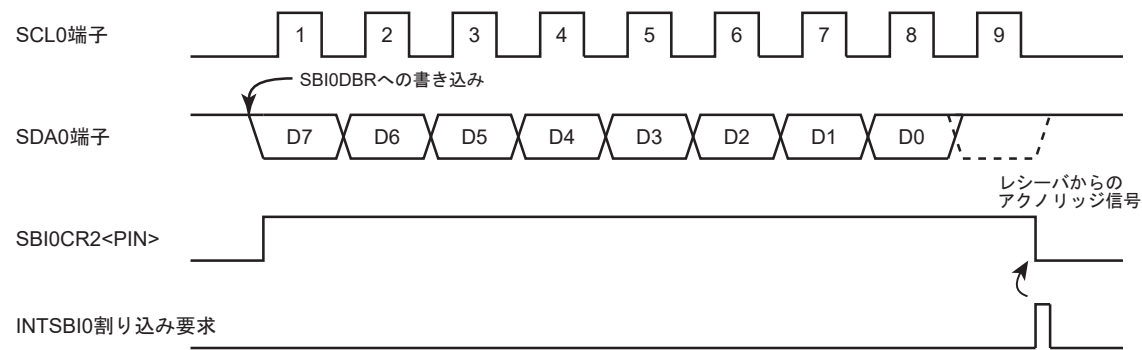
図 20-18 SBI0CR1<BC>=“000”，SBI0CR1<ACK>=“1” の場合
