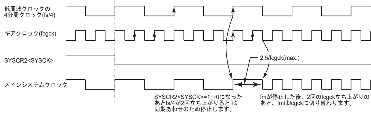
図 2-15 メインシステムクロック (fm)の切り替え (fs/4 から fcgck への切り替え)
