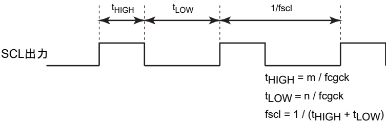
図 20-6 SCL 出力
