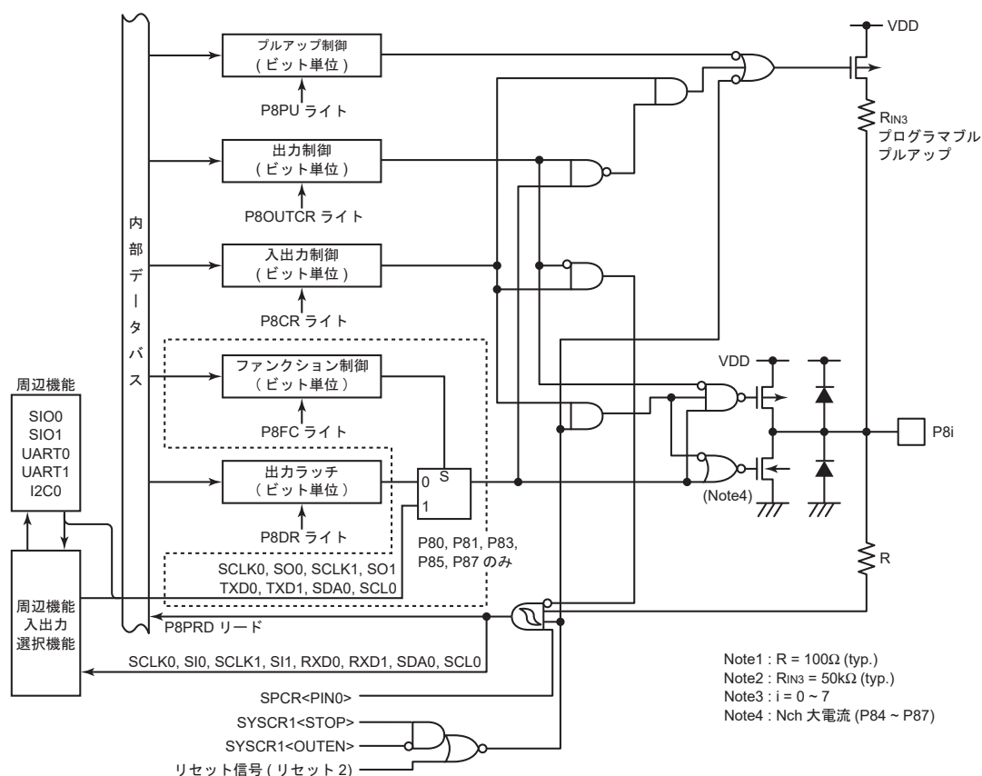
図 8-11 P8 ポート
