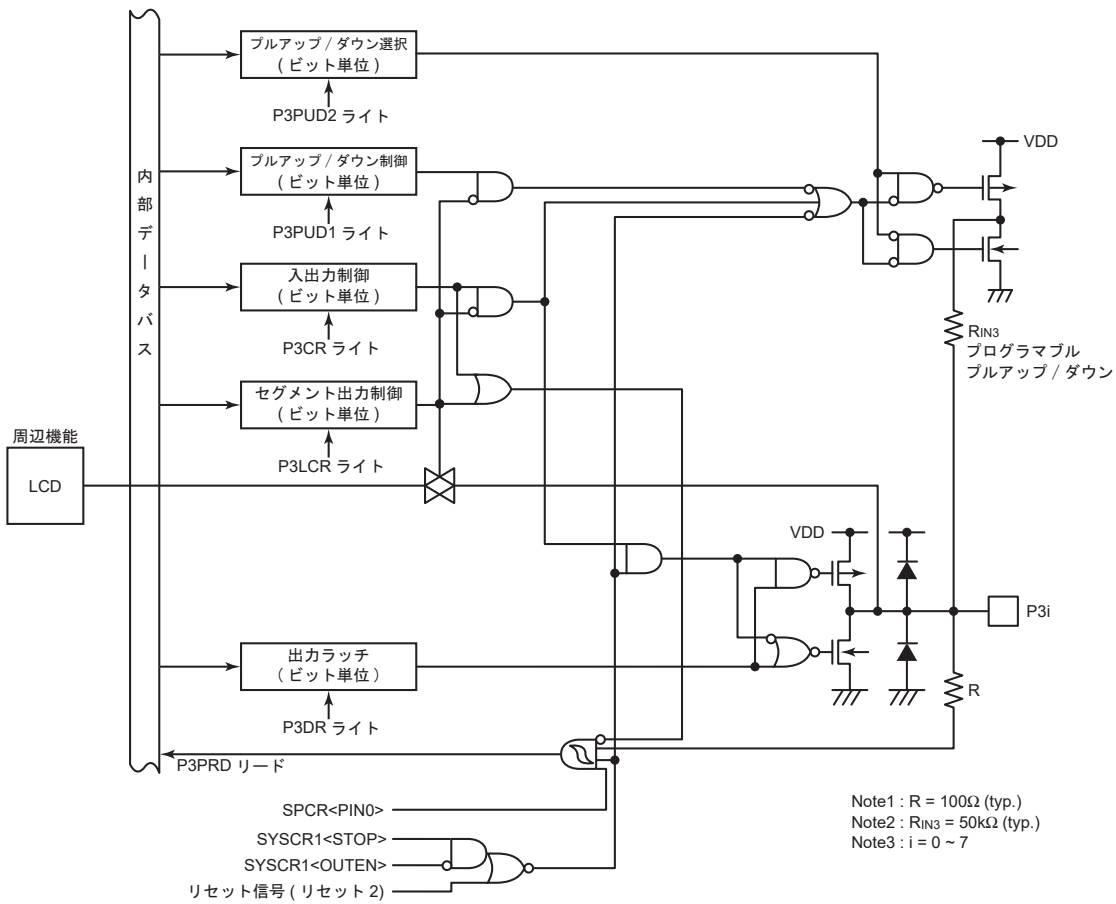
図 8-6 P3 ポート
