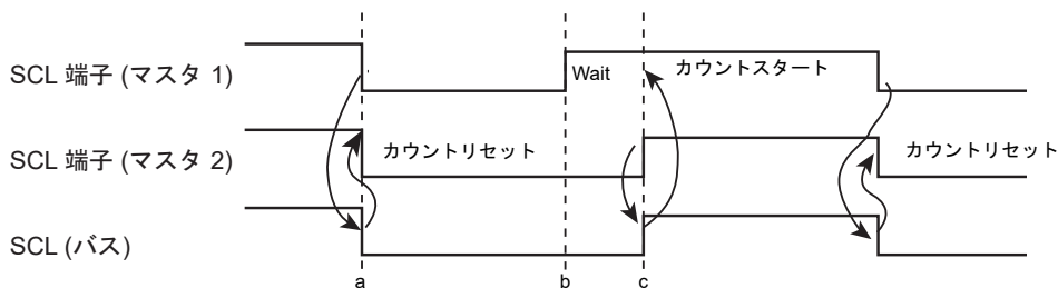
図 20-8 クロック同期化の例
