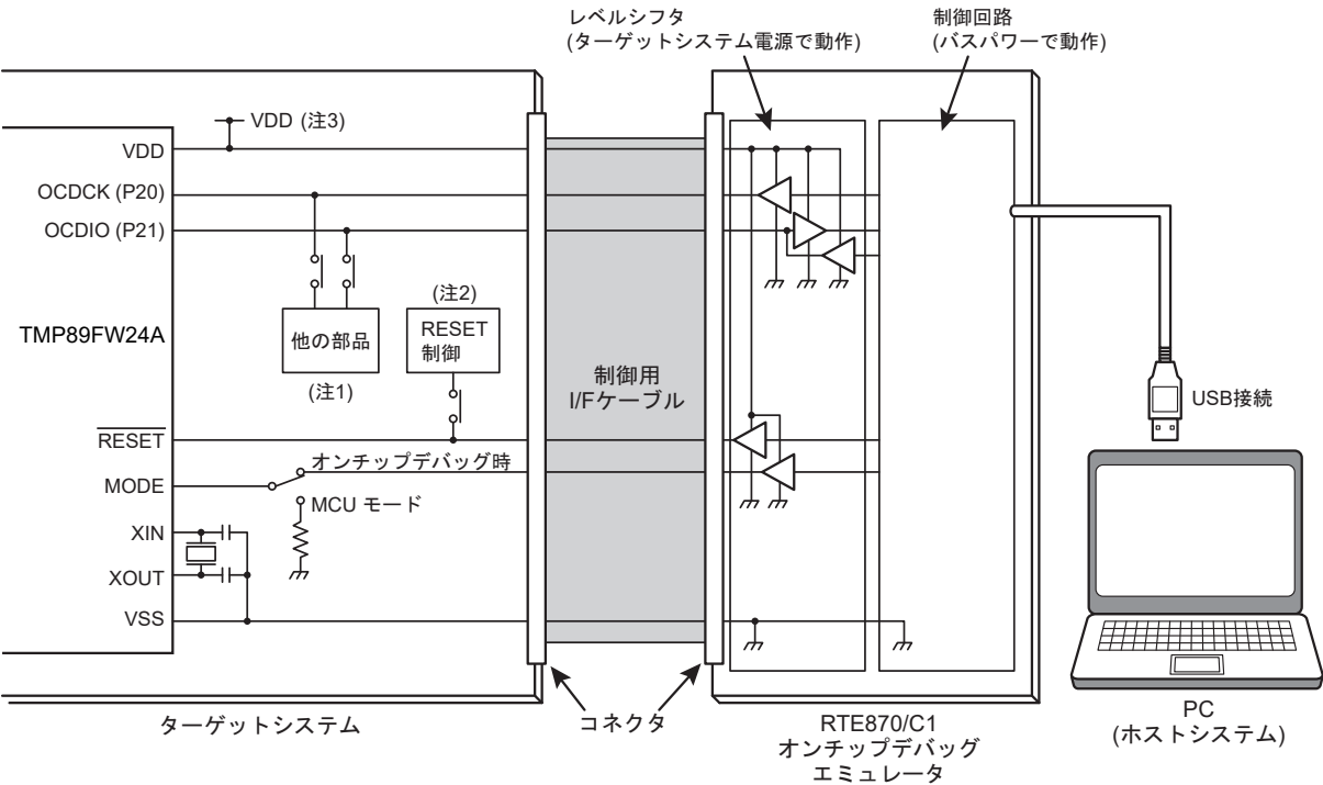
図 27-1 RTE870/C1 オンチップデバッグエミュレータの接続例
