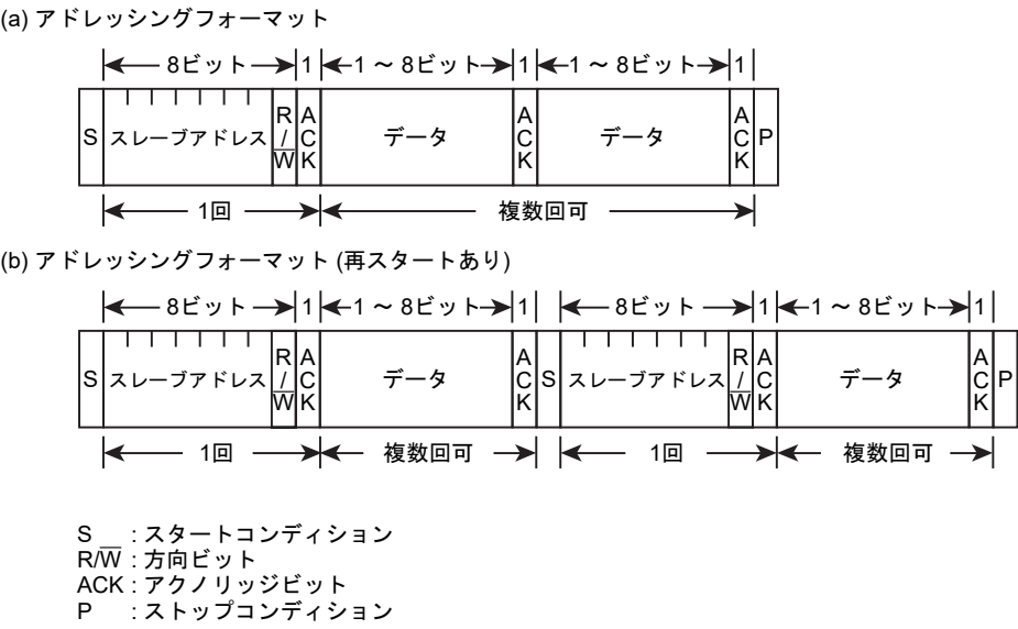
図 20-2 I 2 C バスのデータフォーマット
