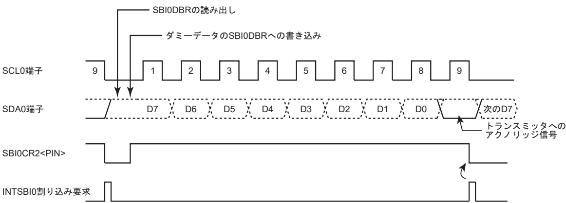
図 20-19 SBI0CR1<BC>=“000”，SBI0CR1<ACK>=“1” の場合
