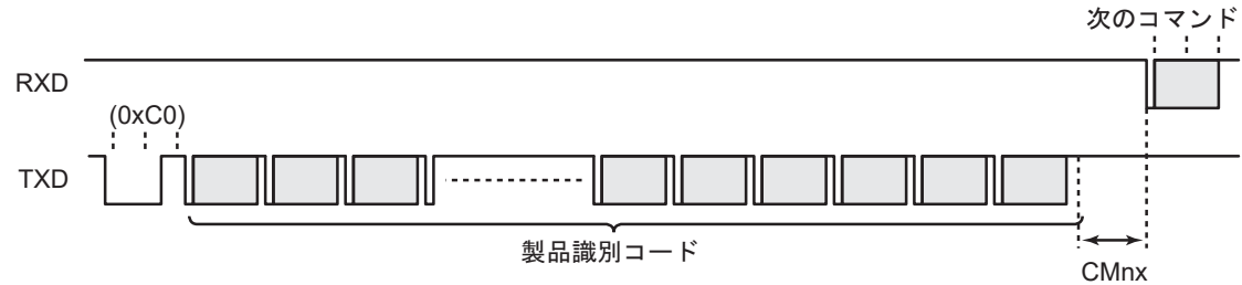
図 26-12 製品識別コード出力コマンド
