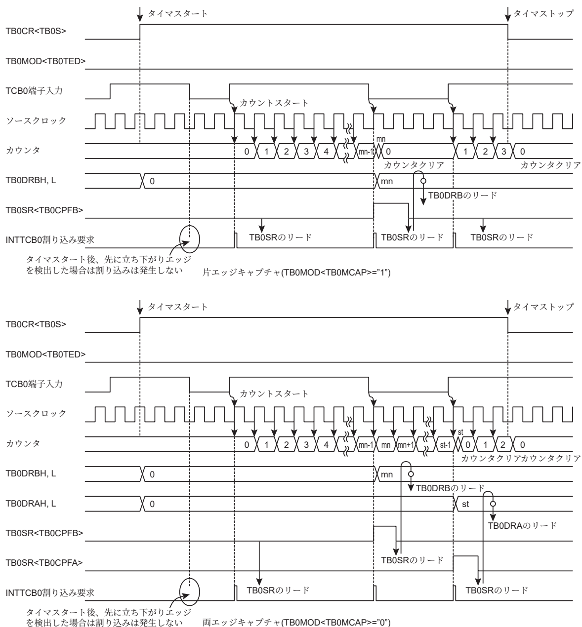
図 14-7 パルス幅測定モードタイミングチャート
