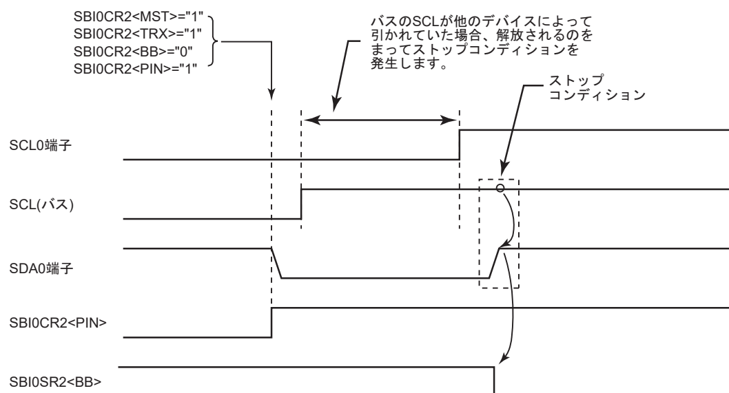
図 20-21 ストップコンディションの発生
