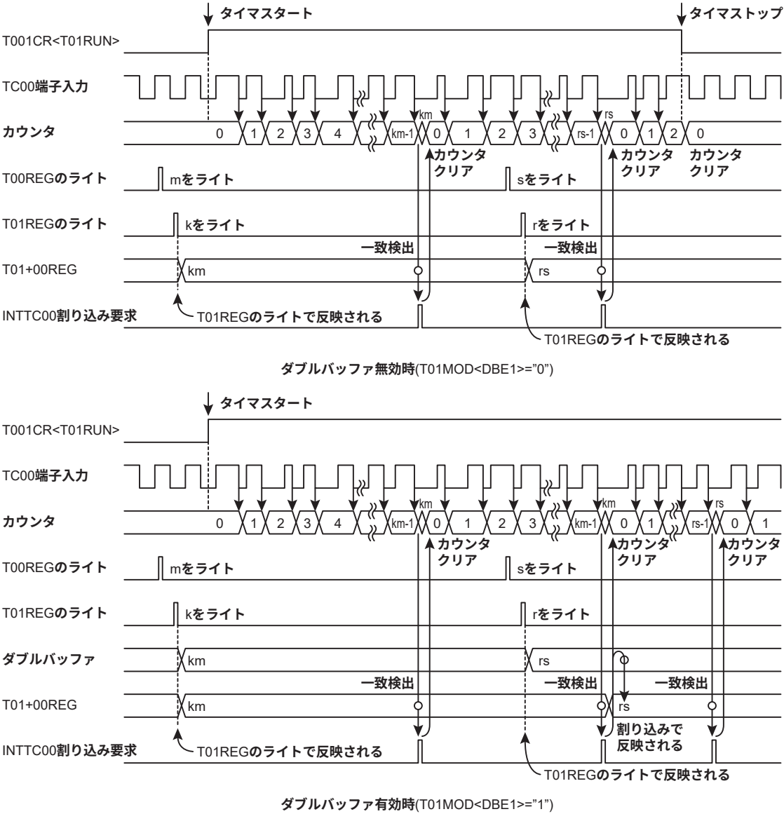
図 16-12 16 ビットイベントカウンタモードタイミングチャート
