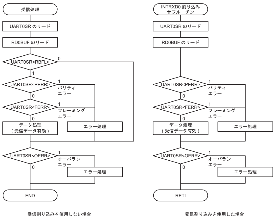
図 18-18 受信処理例
