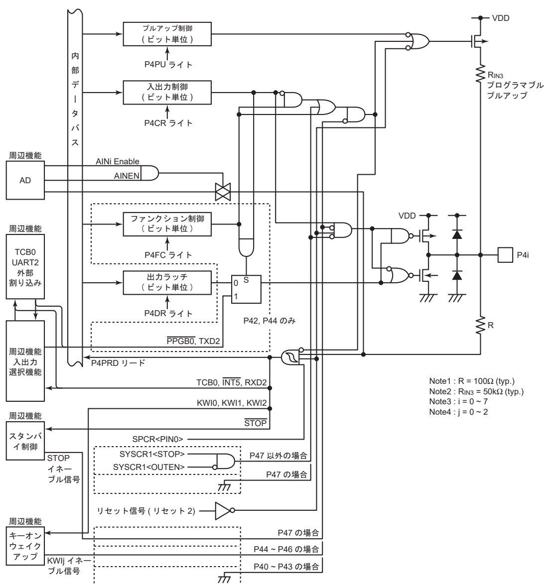
図 8-7 P4 ポート
