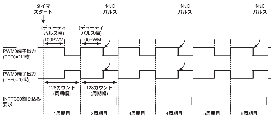
図 16-5 PWM0 パルス出力
