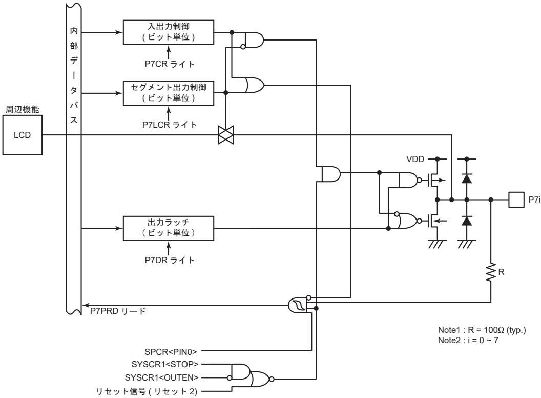
図 8-10 P7 ポート
