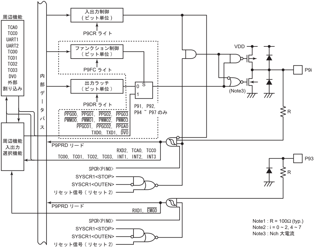
図 8-12 P9 ポート
