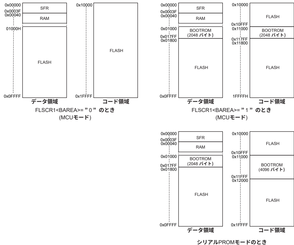
図 26-3 メモリマッピング
