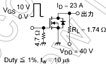
図 6.2.1 スwitching時間の測定回路例
