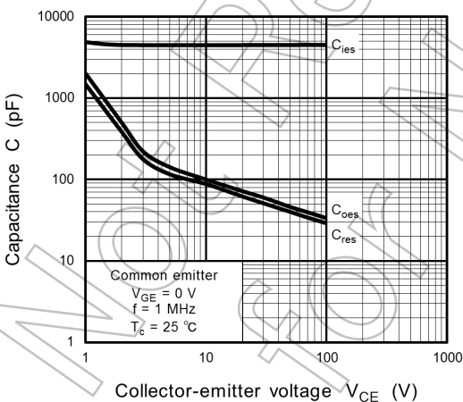
Fig. 8.11 C - V_{CE}
