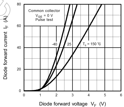
Fig. 8.12 I_F - V_F
