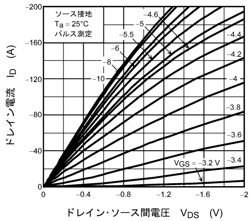
図 9.2 I_D - V_{DS}
