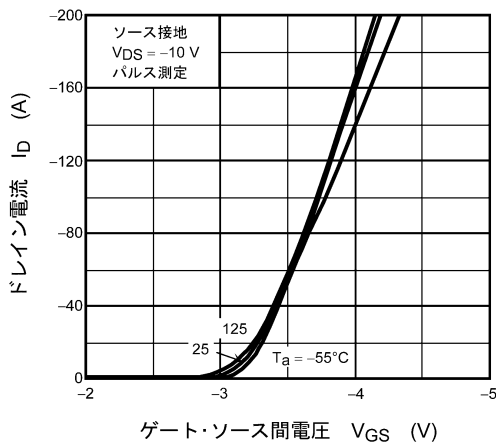
図 9.3 I_D - V_{GS}
