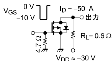
図 6.2.1 スwitchング時間の測定回路
