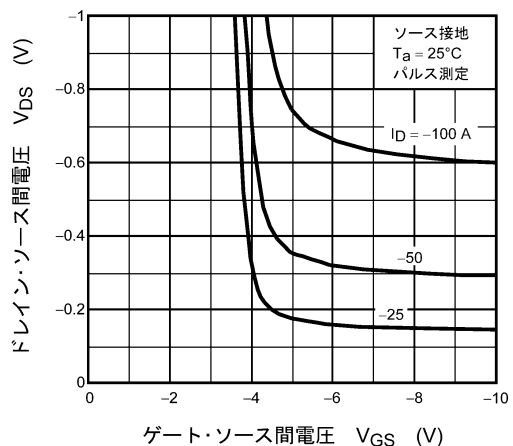
図 9.4 V_{DS} - V_{GS}
