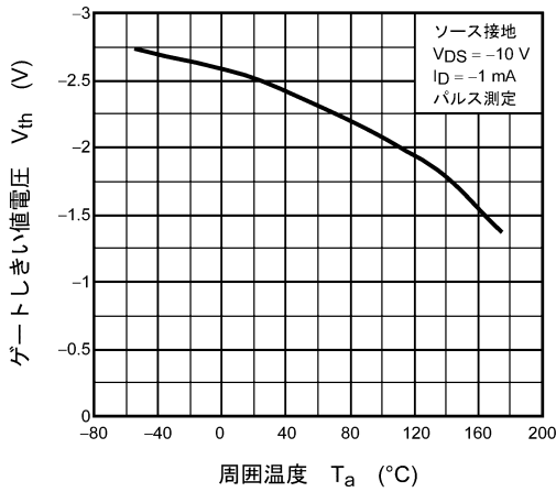
図 9.9 V_{th} - T_a
