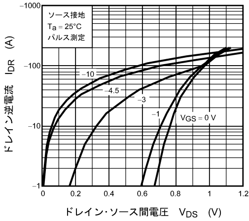
図 9.7 I_{DR} - V_{DS}
