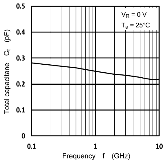
図 8.4 C_t - f
