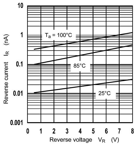
図 8.2 I_R - V_R
