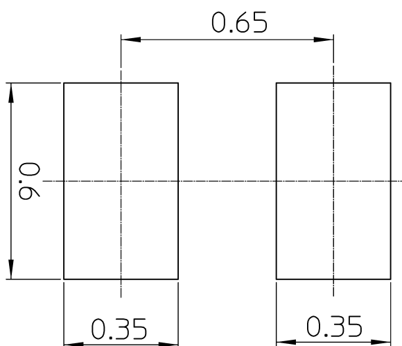
図 7.1 参考パッド寸法 (Unit: mm)
