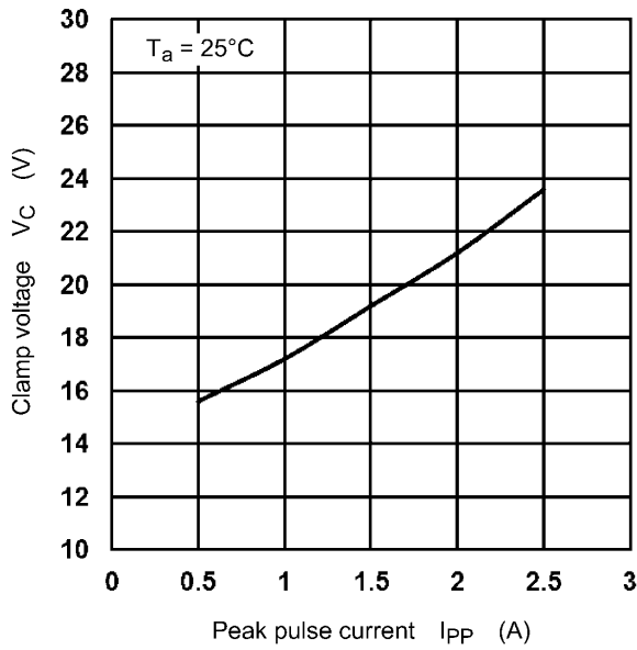
図 9.1 V_C - I_{PP}
