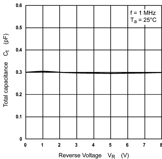
図 8.3 C_t - V_R
