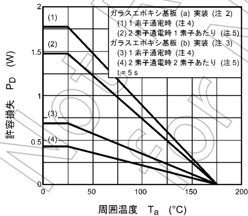
図 8.11 P_D - T_a (注9) (最大値 (保証値))
