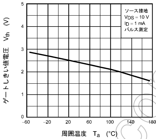
図 8.9 V_{th} - T_a (注9)
