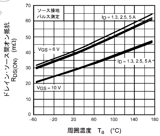
図 8.6 R_{DS(ON)} - T_a (注9)
